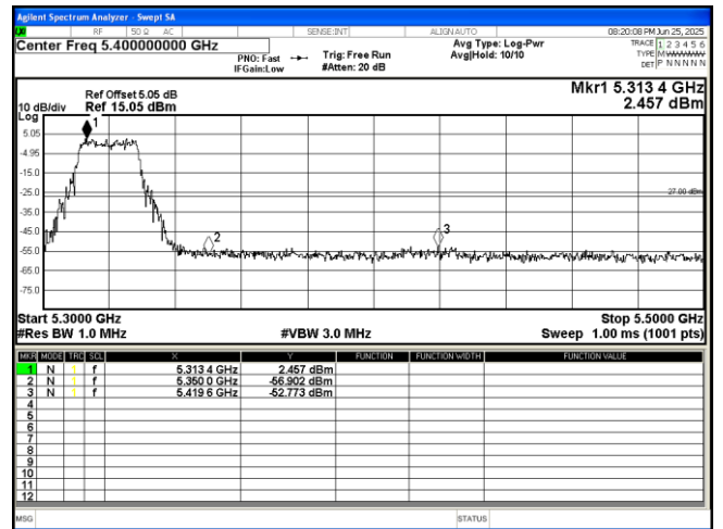
802.11 n20 5320MHz
