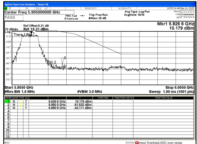
802.11 n20 5825MHz
