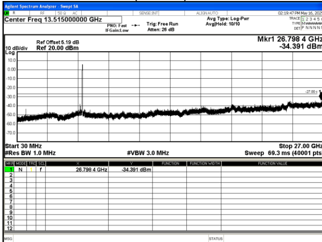
802.11 be(EHT40) 5795MHz
