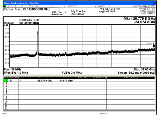
802.11 802.11 be(EHT80) 5210MHz
