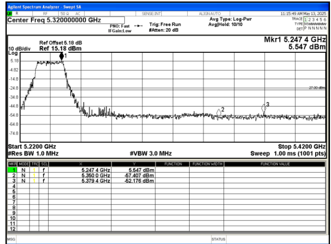
802.11 n20 5240MHz
