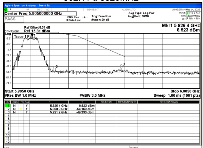
802.11 a 5825MHz
