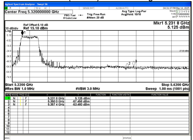
802.11 be(EHT20) 5240MHz
