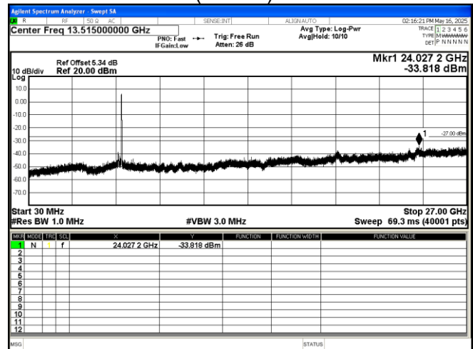
802.11 be(EHT40) 5755MHz
