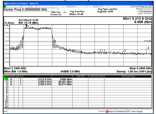
802.11 be(EHT40) 5230MHz
