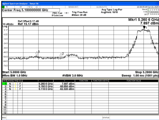
802.11 a 5260MHz
