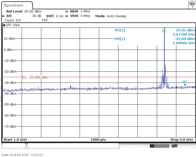
Band41-15MHz-QPSK-41515-1RB#0-Range2:1000~3000MHz
