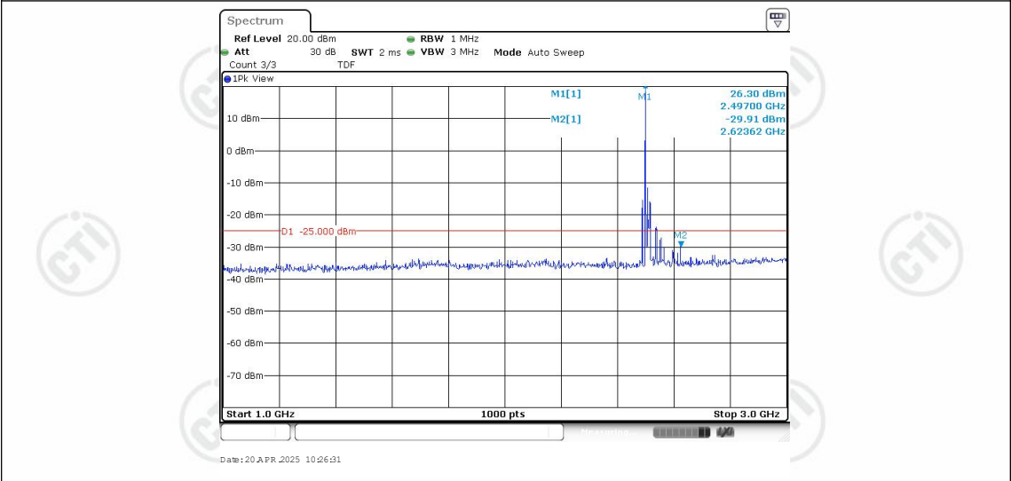
Band41-20MHz-QPSK-39750-1RB#0-Range2:1000~3000MHz
