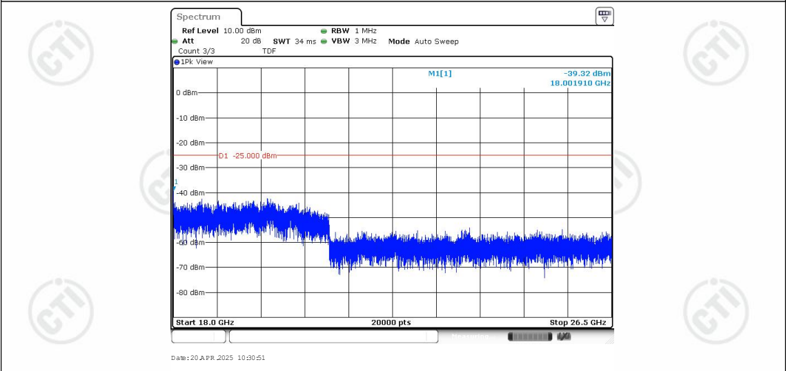
Band41-20MHz-QPSK-41490-1RB#0-Range4:18000~26500MHz
