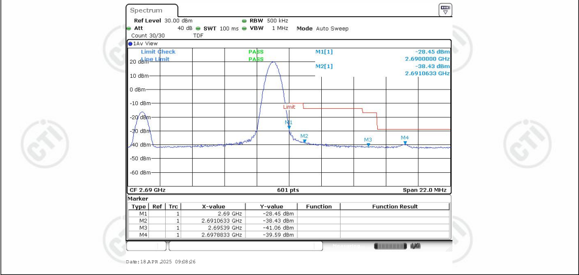
Band41-20MHz-16QAM-41490-1RB#99
