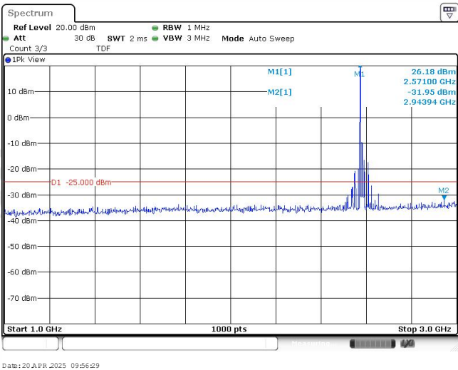
Band38-20MHz-QPSK-37850-1RB#0-Range2:1000~3000MHz
