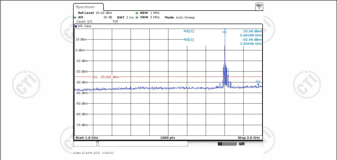
Band38-20MHz-QPSK-38150-1RB#0-Range2:1000~3000MHz
