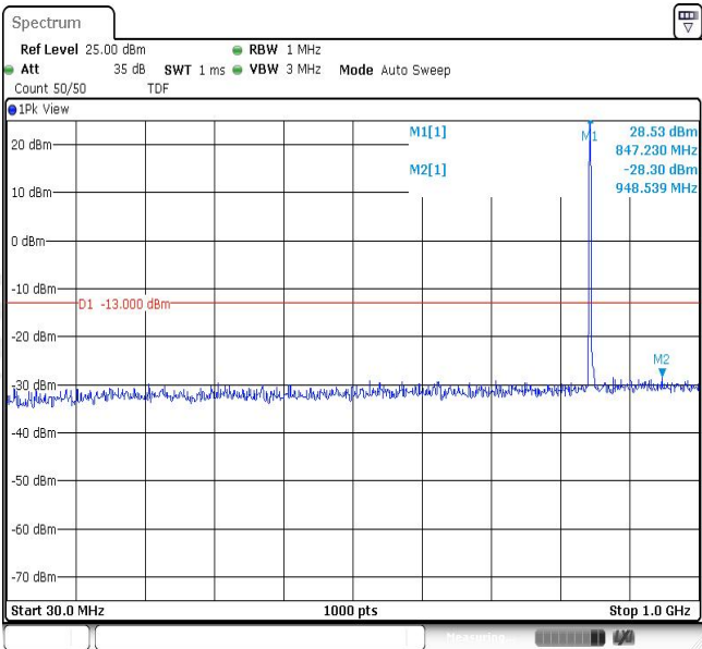
Band26-3MHz-QPSK-27025-1RB#0-Range1:30~1000MHz
