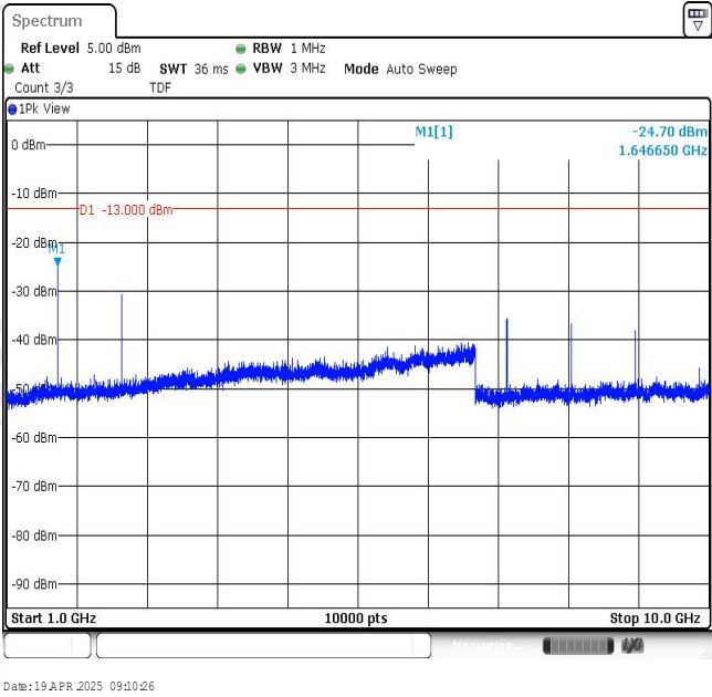
Band26-3MHz-QPSK-26793-1RB#0-Range2:1000~10000MHz
