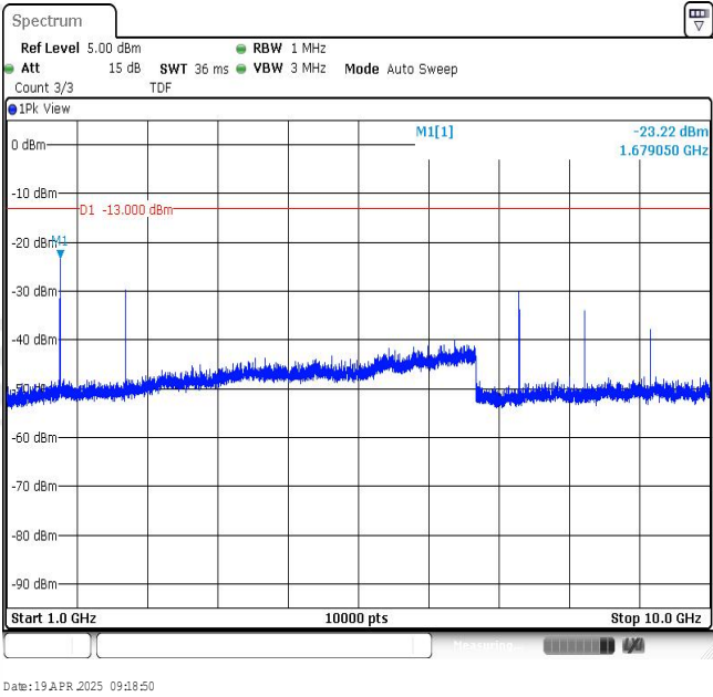
Band26-10MHz-QPSK-26990-1RB#0-Range2:1000~10000MHz
