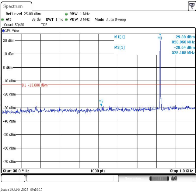
Band26-3MHz-QPSK-26793-1RB#0-Range1:30~1000MHz
