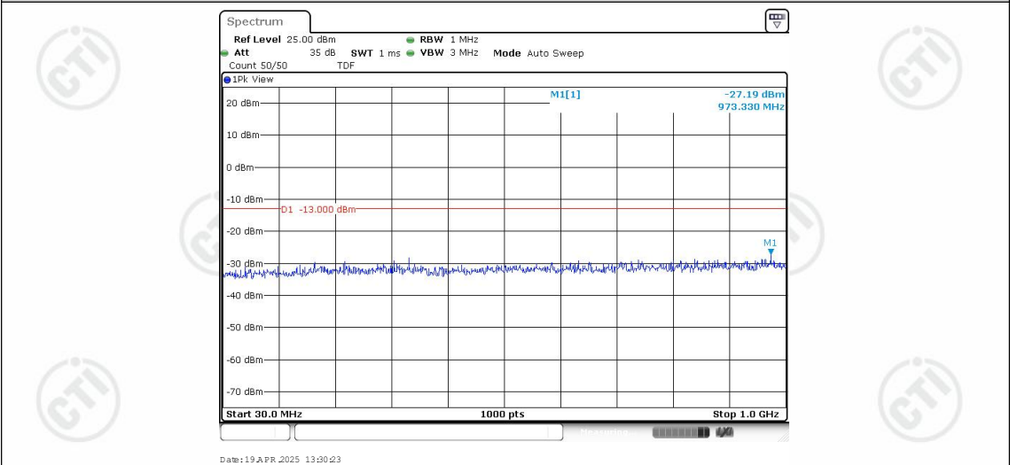
Band25-20MHz-QPSK-26365-1RB#0-Range1:30~1000MHz
