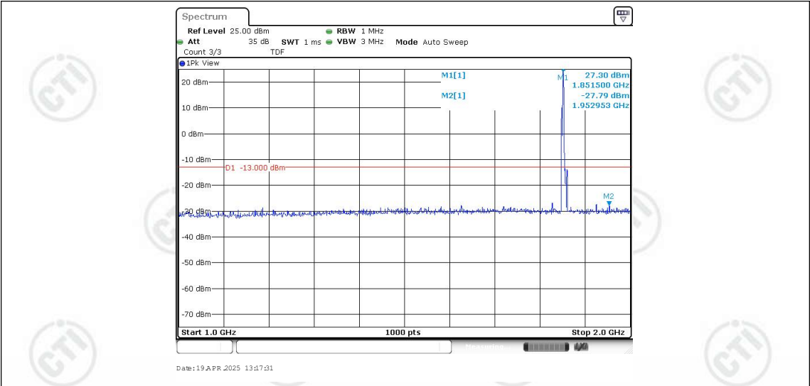
Band25-5MHz-QPSK-26065-1RB#0-Range2:1000~2000MHz
