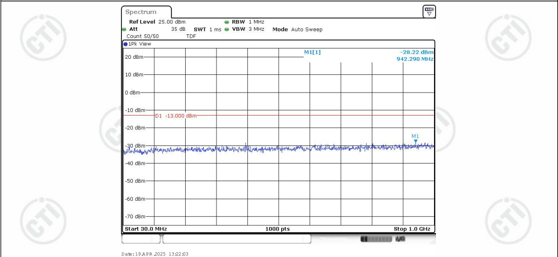
Band25-10MHz-QPSK-26365-1RB#0-Range1:30~1000MHz
