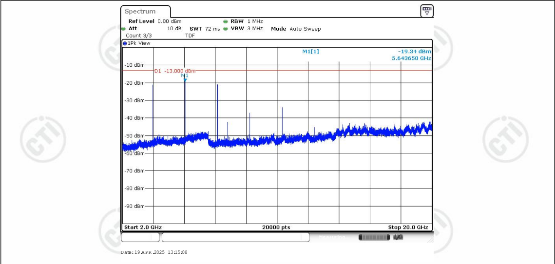
Band25-3MHz-QPSK-26365-1RB#0-Range3:2000~20000MHz
