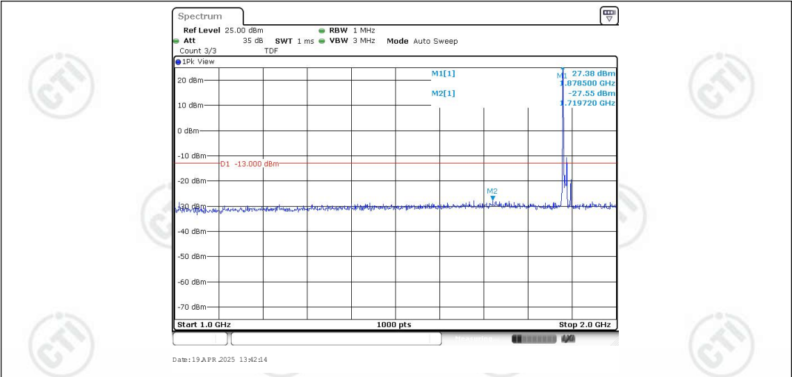
Band25-10MHz-16QAM-26365-1RB#0-Range2:1000~2000MHz
