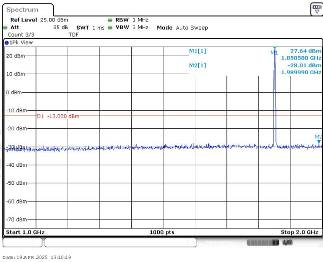
Band25-1.4MHz-QPSK-26047-1RB#0-Range2:1000~2000MHz
