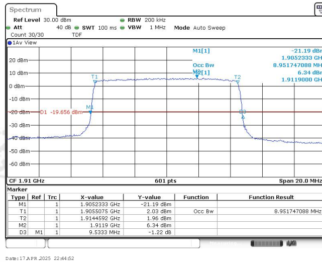
Band25-10MHz-QPSK-26640-50RB#0-8.952
