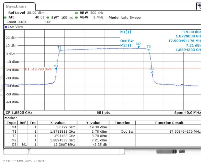
Band25-20MHz-QPSK-26365-100RB#0-17.903
