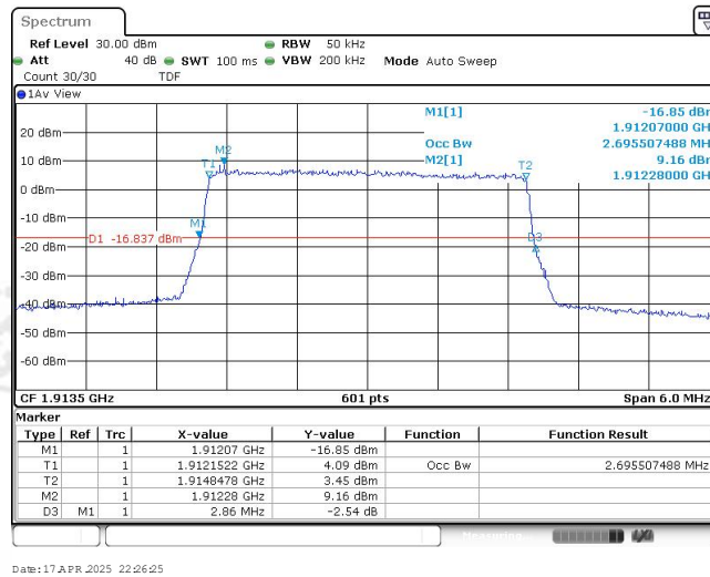
Band25-3MHz-QPSK-26675-15RB#0-2.696
