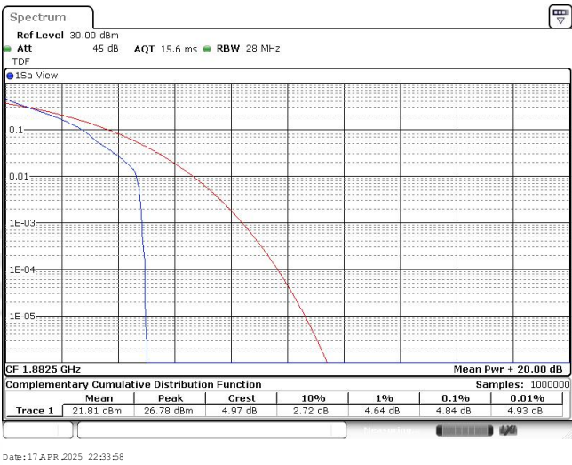
Band25-5MHz-QPSK-26365-1RB#0
