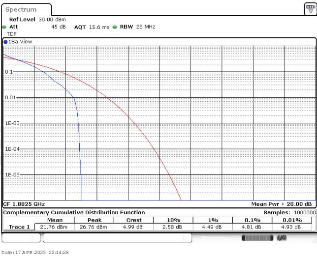
Band25-1.4MHz-QPSK-26365-1RB#0
