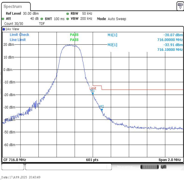
Band12-3MHz-QPSK-23165-1RB#14
