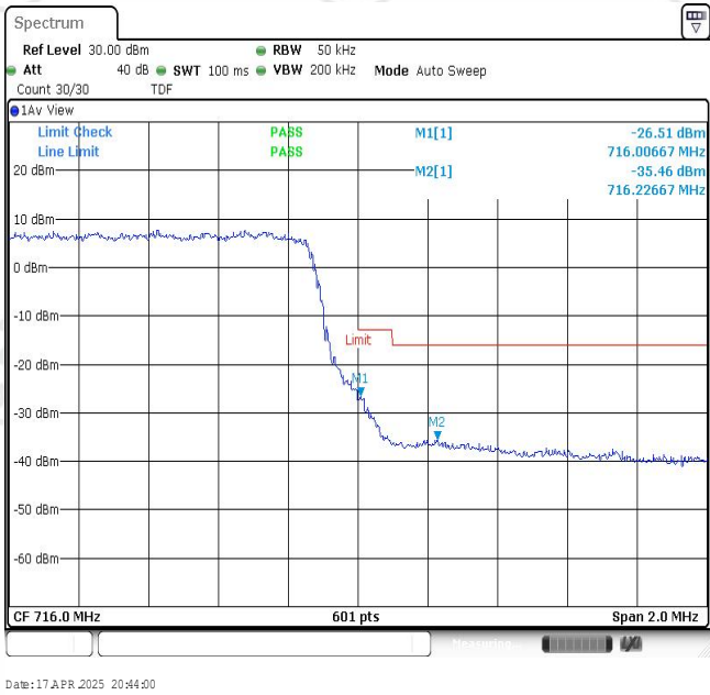
Band12-3MHz-QPSK-23165-15RB#0
