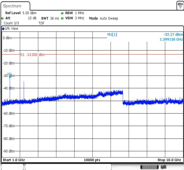
Band12-1.4MHz-QPSK-23017-1RB#0-Range2:1000~10000MHz
