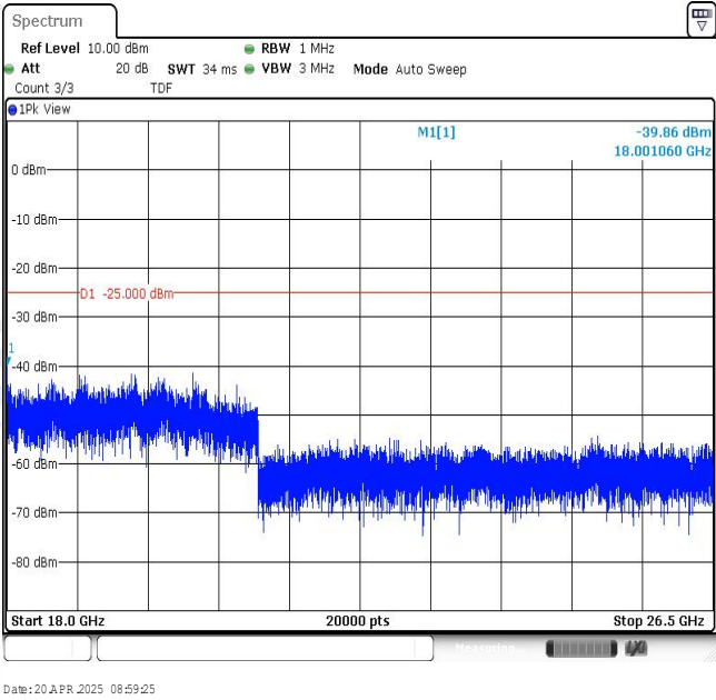
Band7-5MHz-QPSK-20775-1RB#0-Range4:18000~26500MHz
