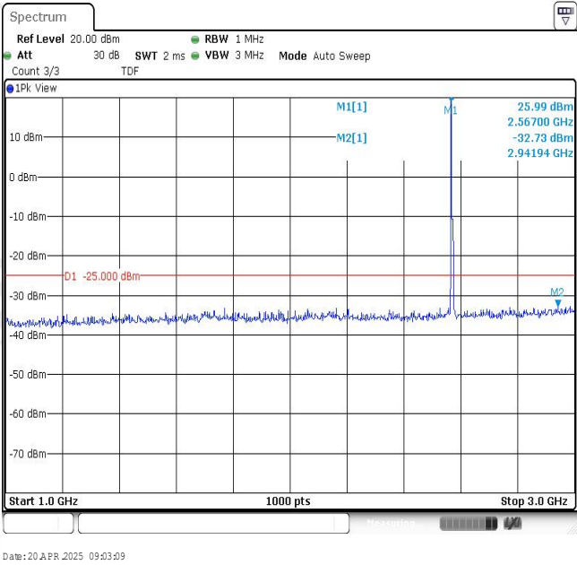
Band7-5MHz-QPSK-21425-1RB#0-Range2:1000~3000MHz
