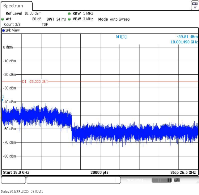
Band7-5MHz-QPSK-21425-1RB#0-Range4:18000~26500MHz
