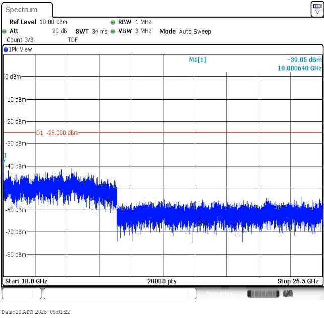
Band7-5MHz-QPSK-21100-1RB#0-Range4:18000~26500MHz
