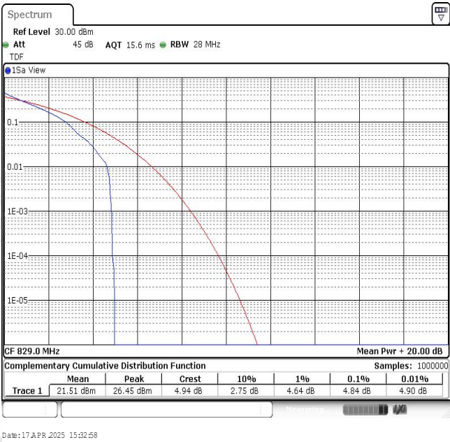
Band5-10MHz-QPSK-20450-1RB#0
