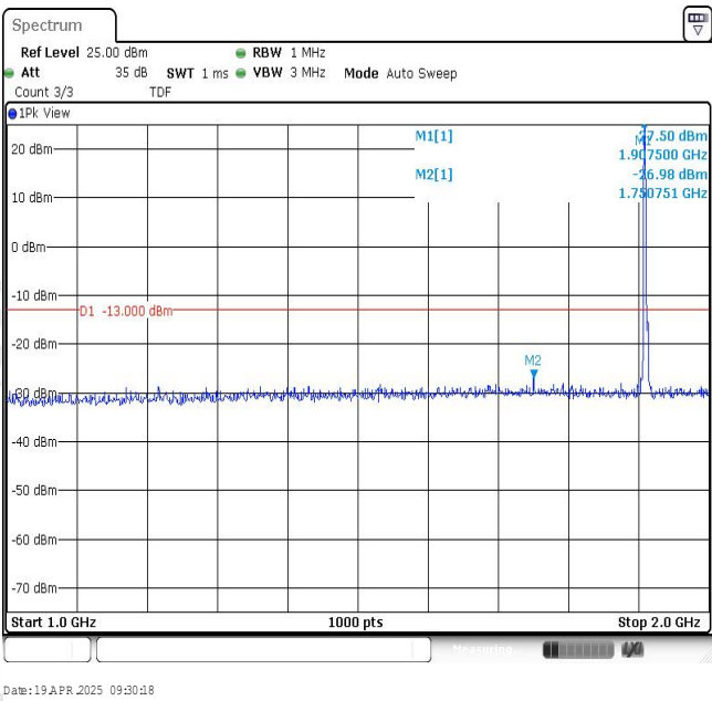
Band2-3MHz-QPSK-19185-1RB#0-Range2:1000~2000MHz
