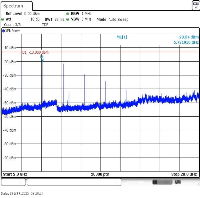
Band2-3MHz-QPSK-19185-1RB#0-Range3:2000~20000MHz
