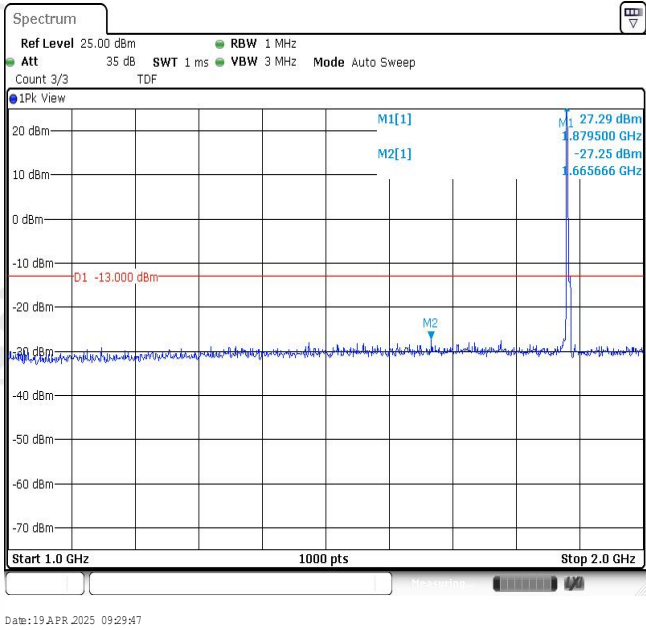
Band2-3MHz-QPSK-18900-1RB#0-Range2:1000~2000MHz
