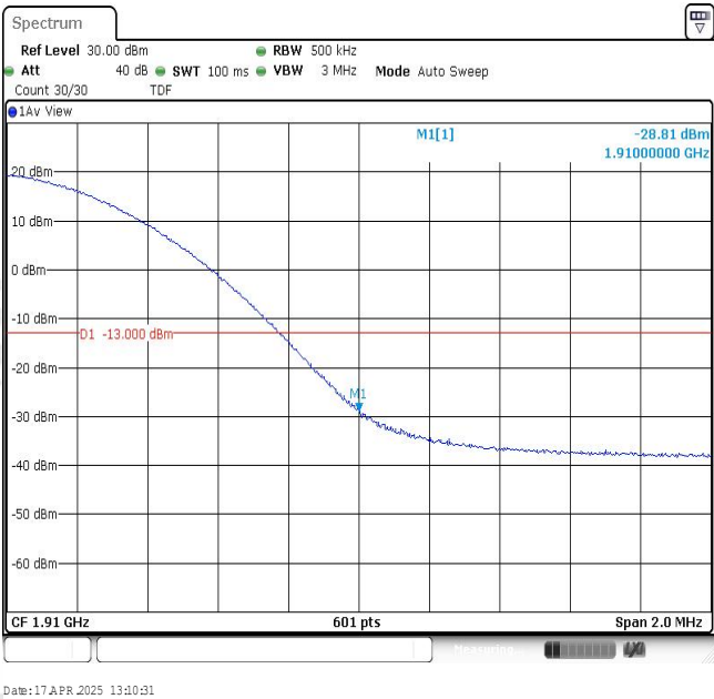
Band2-20MHz-16QAM-19100-1RB#99
