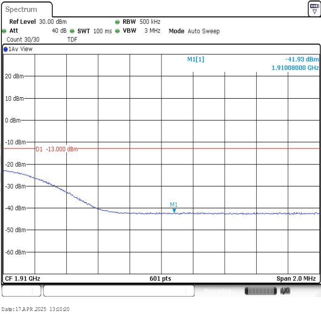
Band2-20MHz-16QAM-19100-1RB#0
