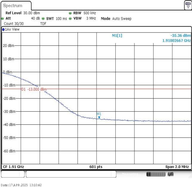
Band2-20MHz-16QAM-19100-100RB#0
