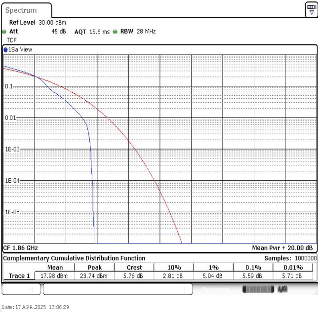
Band2-20MHz-16QAM-18700-1RB#0
