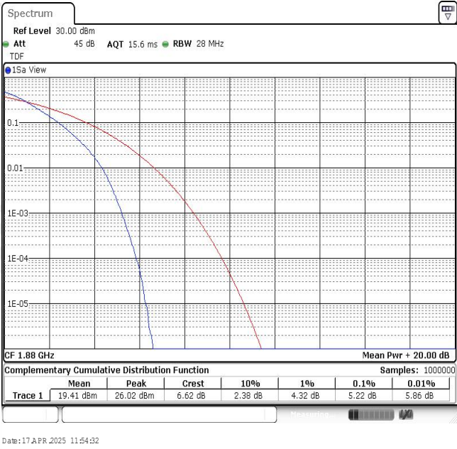
Band2-20MHz-QPSK-18900-100RB#0
