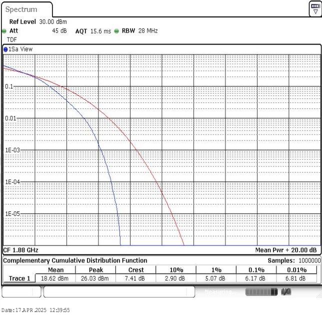
Band2-10MHz-16QAM-18900-50RB#0
