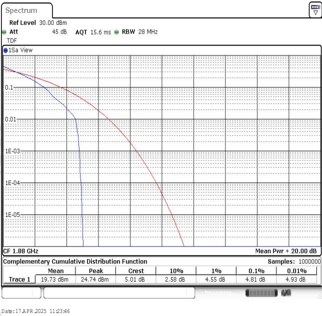
Band2-10MHz-QPSK-18900-1RB#0
