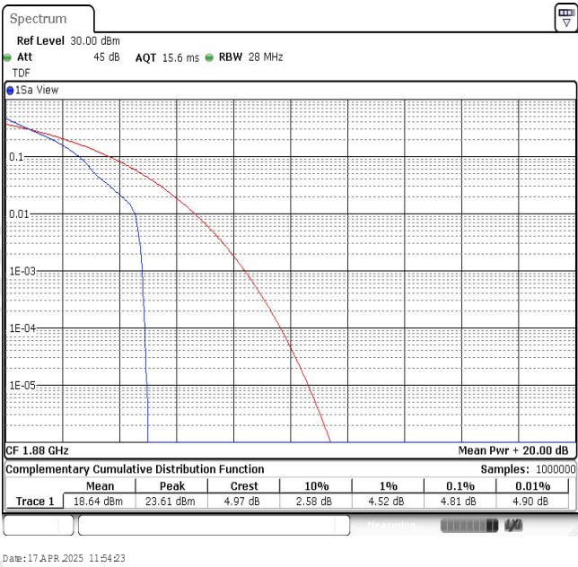
Band2-20MHz-QPSK-18900-1RB#0
