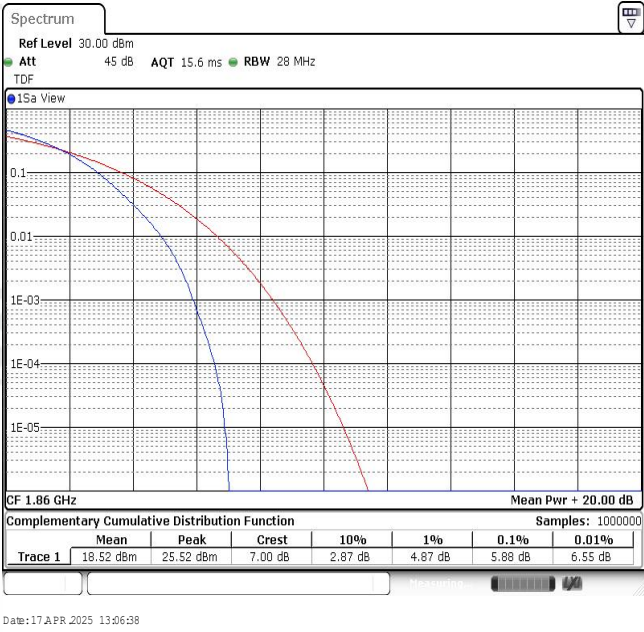
Band2-20MHz-16QAM-18700-100RB#0
