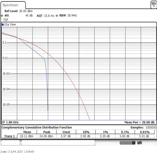
Band2-20MHz-16QAM-18900-1RB#0
