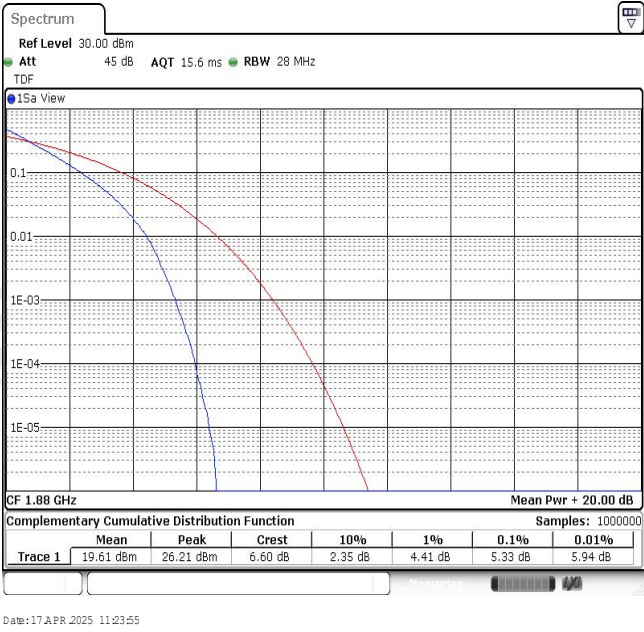
Band2-10MHz-QPSK-18900-50RB#0
