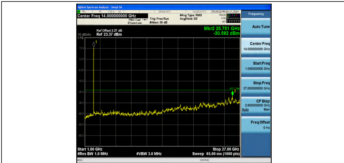
Band41-20MHz-QPSK-39750-1RB#0-Range2:1000~27000MHz
