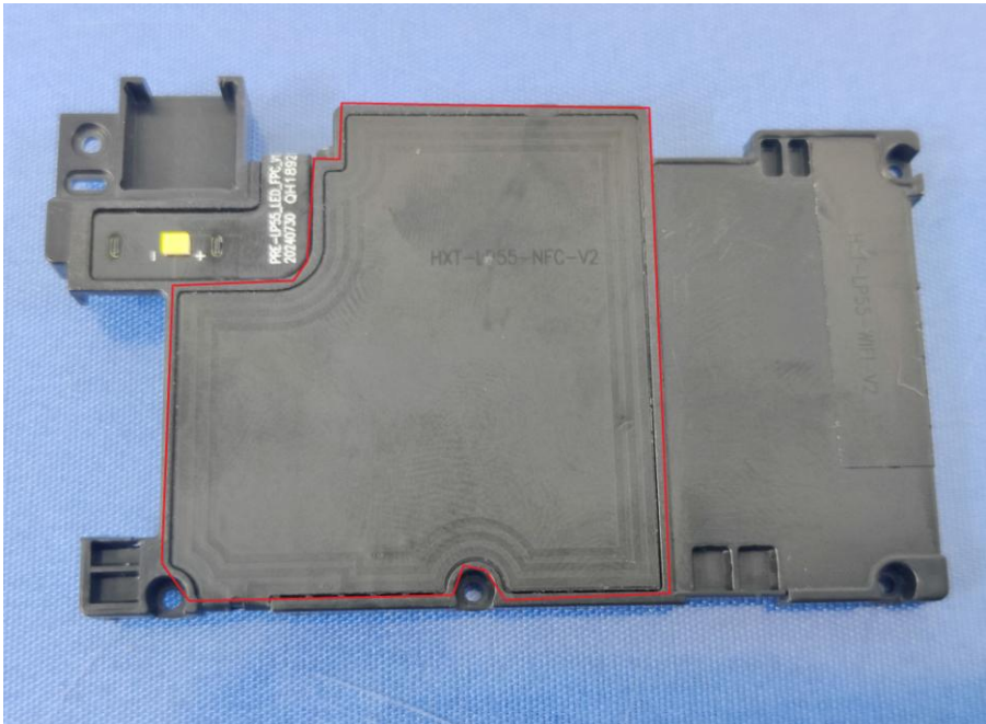
NFC ANT
