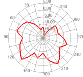
2470.000MHz E1
