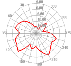
2410.000MHz E1
