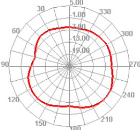
2470.000MHz H
