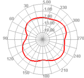
2410.000MHz H
