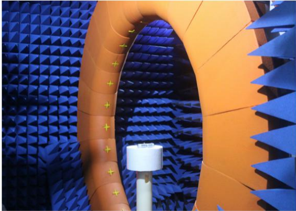
24 探头微波暗室
