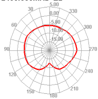
2450.000MHz H
