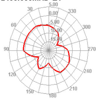
2450.000MHz
