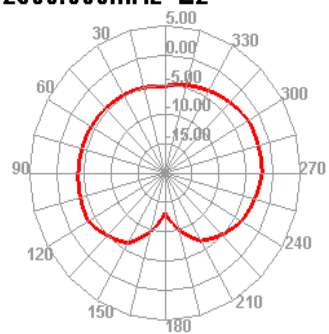
2500.000MHz E2
