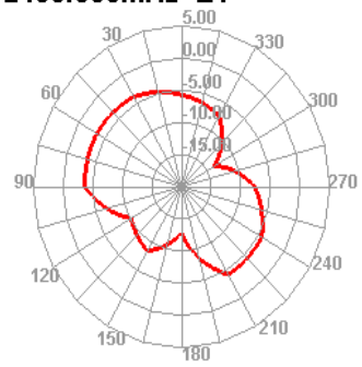
2450.000MHz E1
