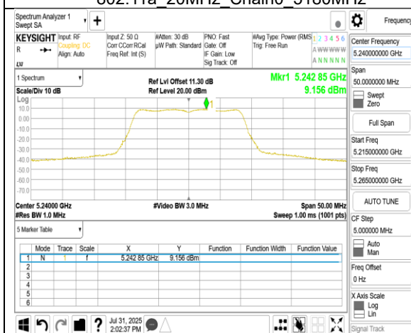
802.11a 20MHz Chain0 5240MHz
