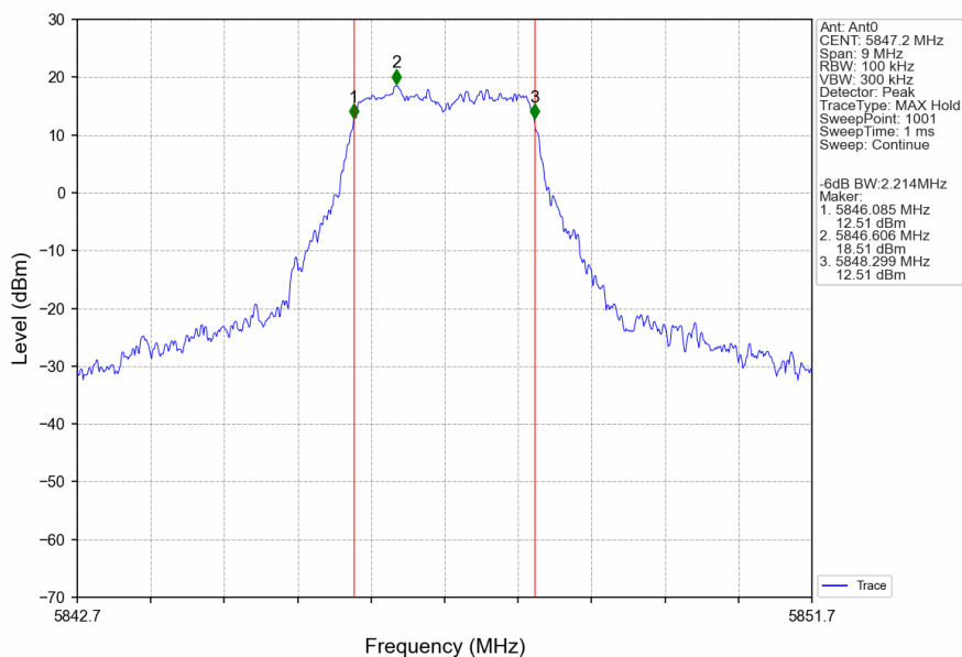
3M_HCH_5847.2MHz_Ant0_NTNV
