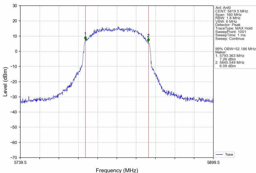
60M_HCH_5819.5MHz_Ant0_NTNV
