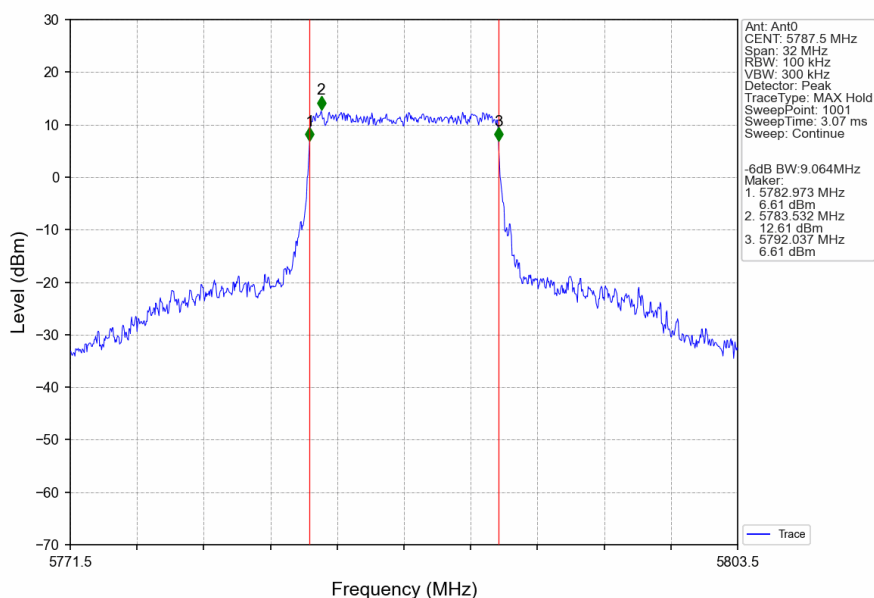
10M_MCH_5787.5MHz_Ant0_NTNV
