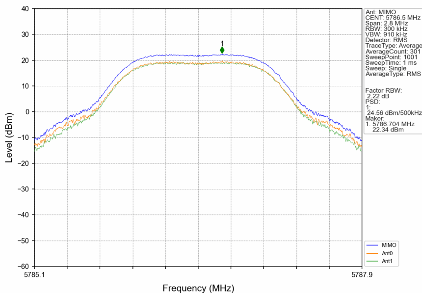
1.4M_MCH_5786.5MHz_MIMO_NTNV
