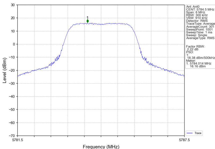
3M_MCH_5784.5MHz_Ant0_NTNV
