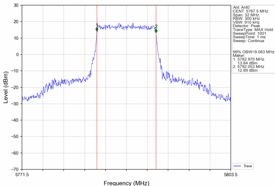
10M_MCH_5787.5MHz_Ant0_NTNV
