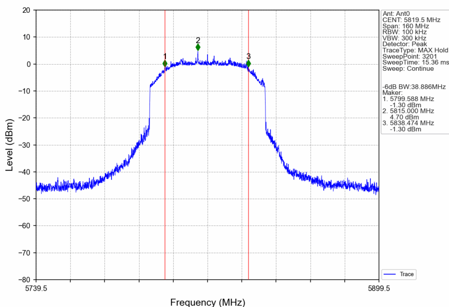
60M_HCH_5819.5MHz_Ant0_NTNV
