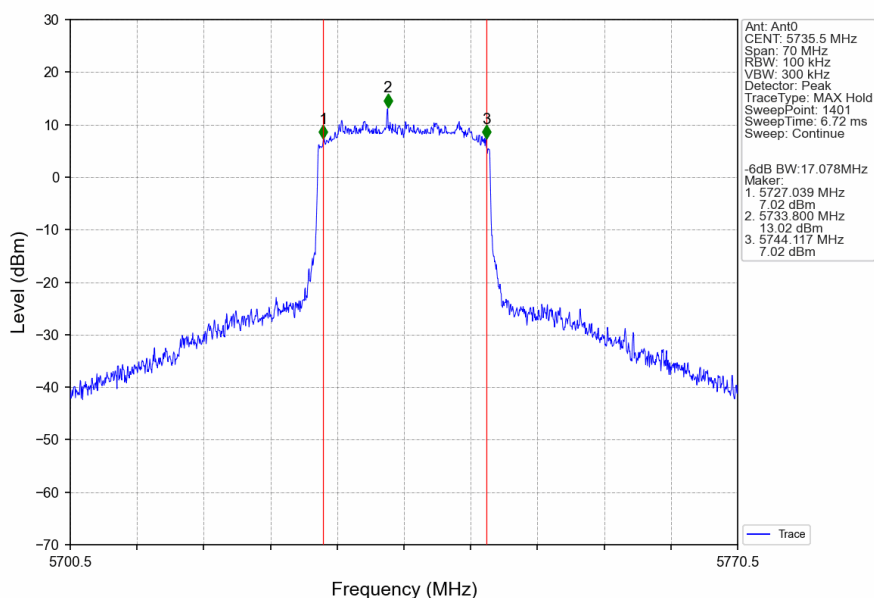
20M_LCH_5735.5MHz_Ant0_NTNV
