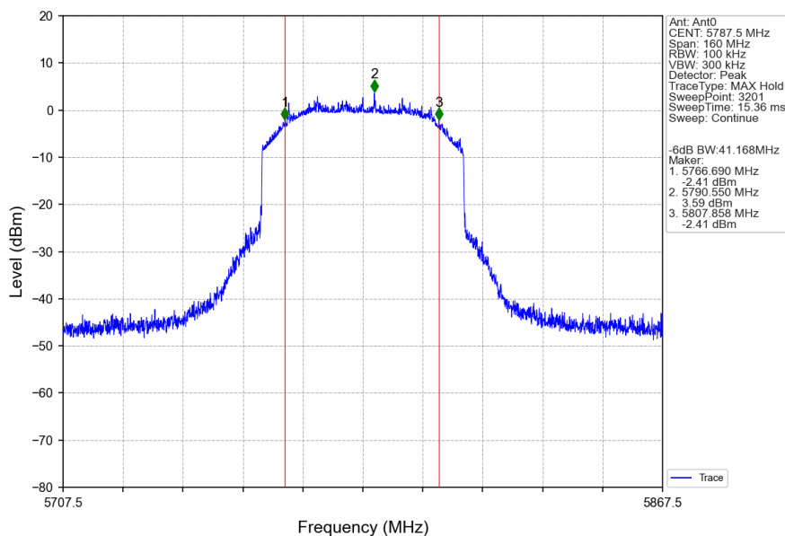
60M_MCH_5787.5MHz_Ant0_NTNV
