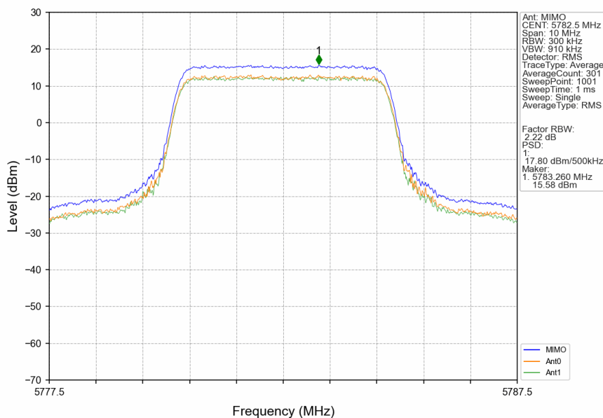
5M_MCH_5782.5MHz_MIMO_NTNV
