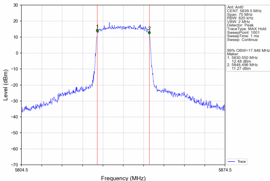
20M_HCH_5839.5MHz_Ant0_NTNV
