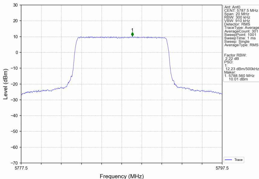
10M_MCH_5787.5MHz_Ant0_NTNV
