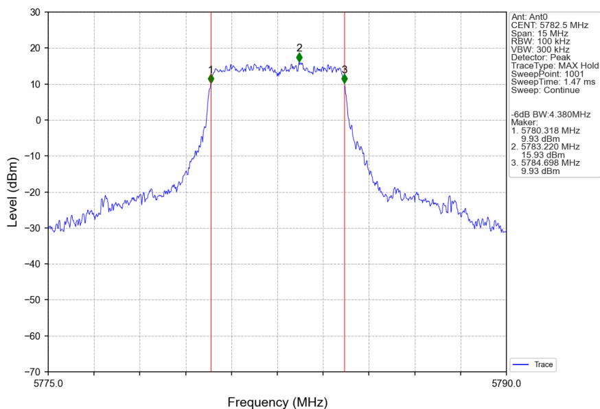
5M_MCH_5782.5MHz_Ant0_NTNV
