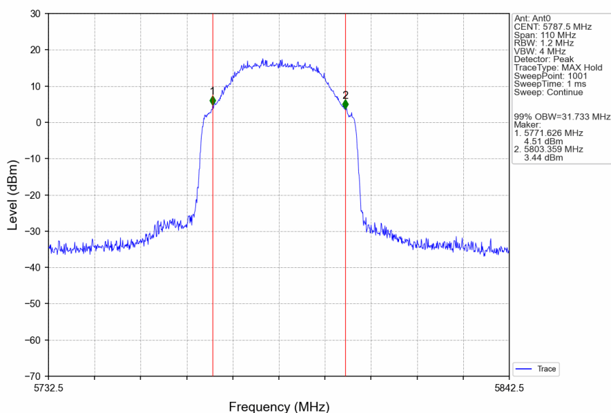
40M_MCH_5787.5MHz_Ant0_NTNV
