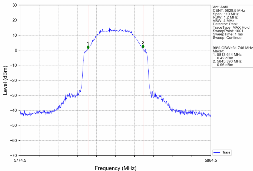
40M_HCH_5829.5MHz_Ant0_NTNV
