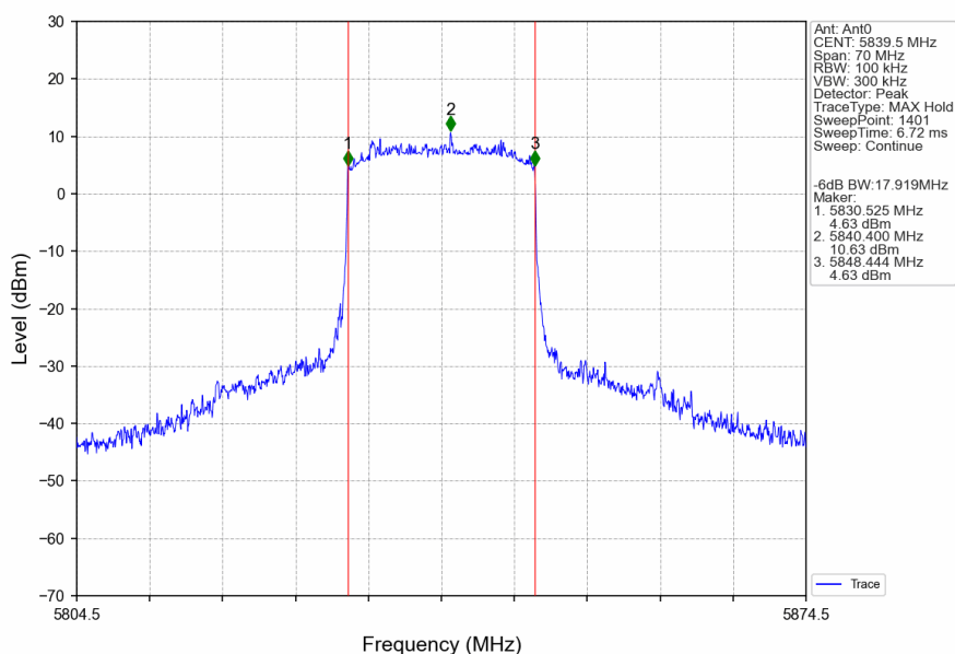
20M_HCH_5839.5MHz_Ant0_NTNV
