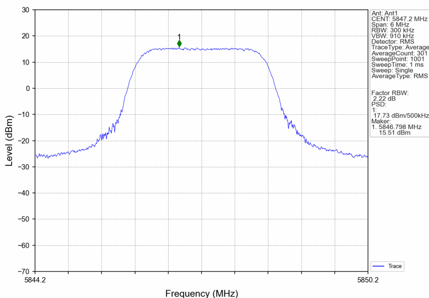
3M_HCH_5847.2MHz_Ant1_NTNV
