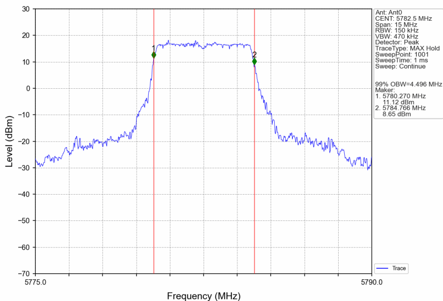
5M_MCH_5782.5MHz_Ant0_NTNV
