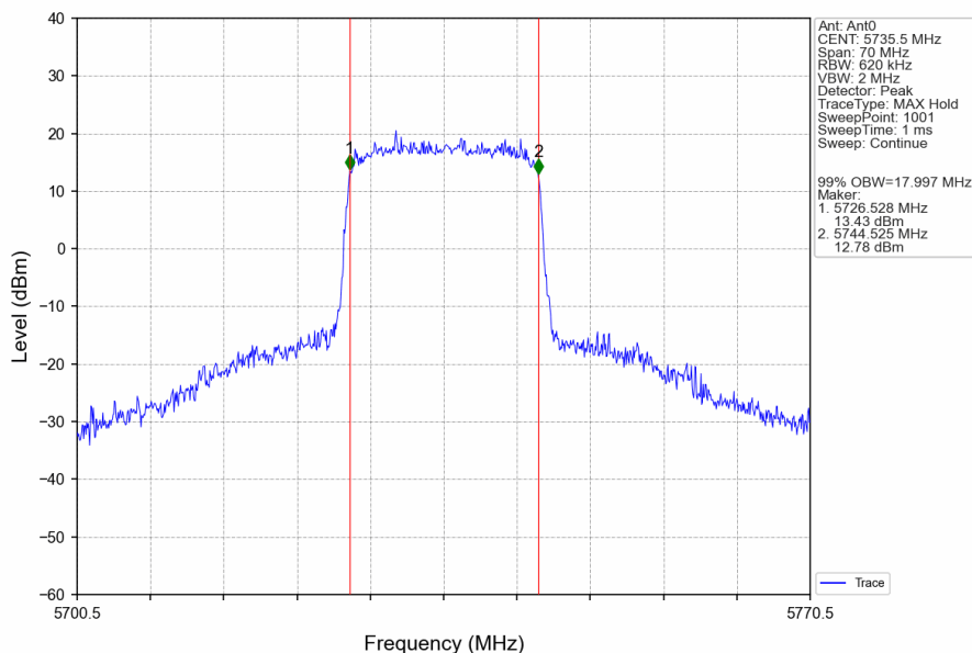
20M_LCH_5735.5MHz_Ant0_NTNV
