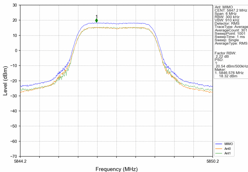
3M_HCH_5847.2MHz_MIMO_NTNV
