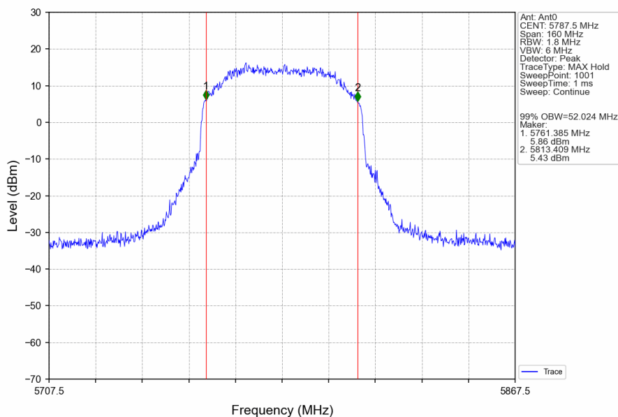
60M_MCH_5787.5MHz_Ant0_NTNV
