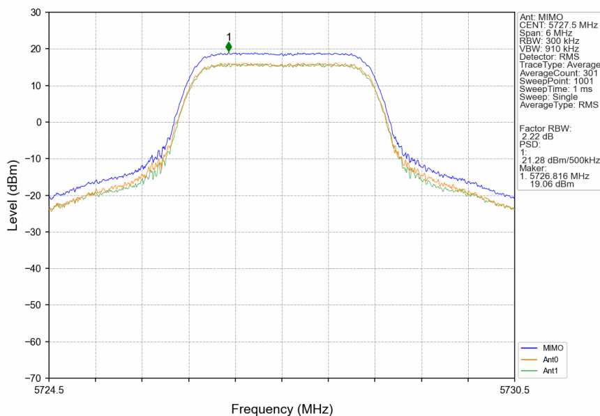
3M_LCH_5727.5MHz_MIMO_NTNV
