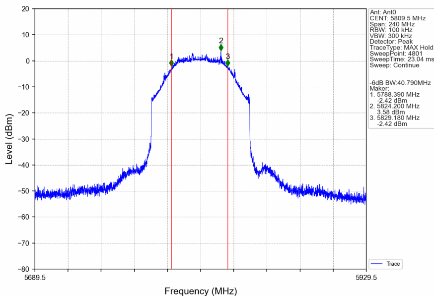
80M_HCH_5809.5MHz_Ant0_NTNV
