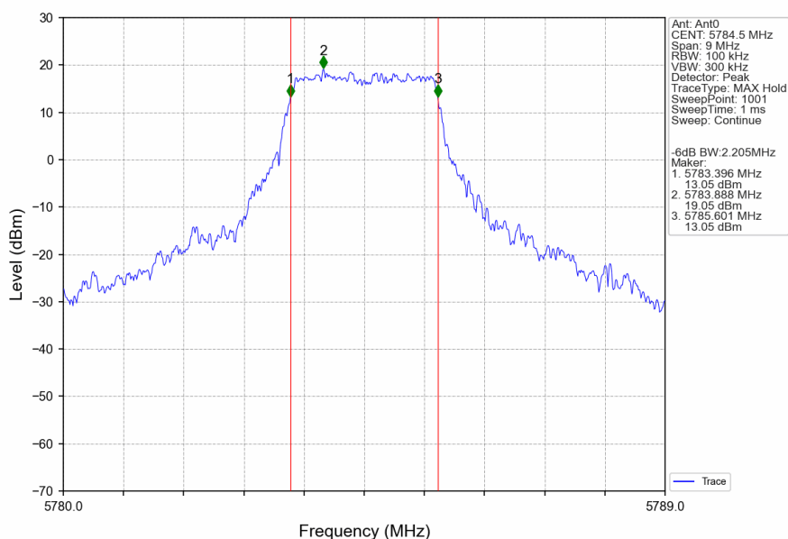
3M_MCH_5784.5MHz_Ant0_NTNV
