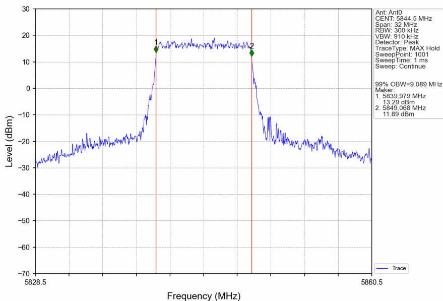
10M_HCH_5844.5MHz_Ant0_NTNV
