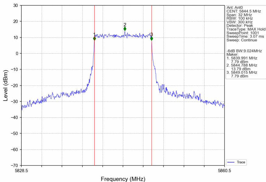
10M_HCH_5844.5MHz_Ant0_NTNV
