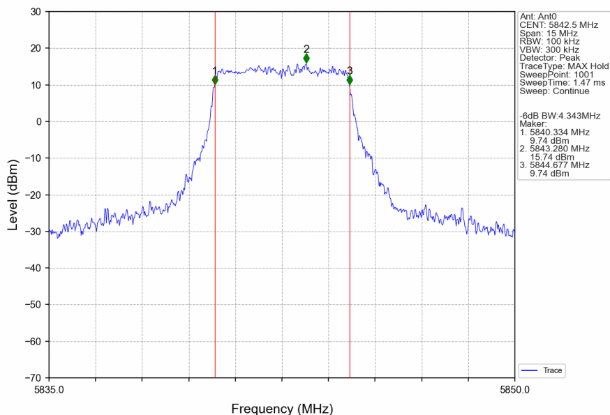
5M_HCH_5842.5MHz_Ant0_NTNV
