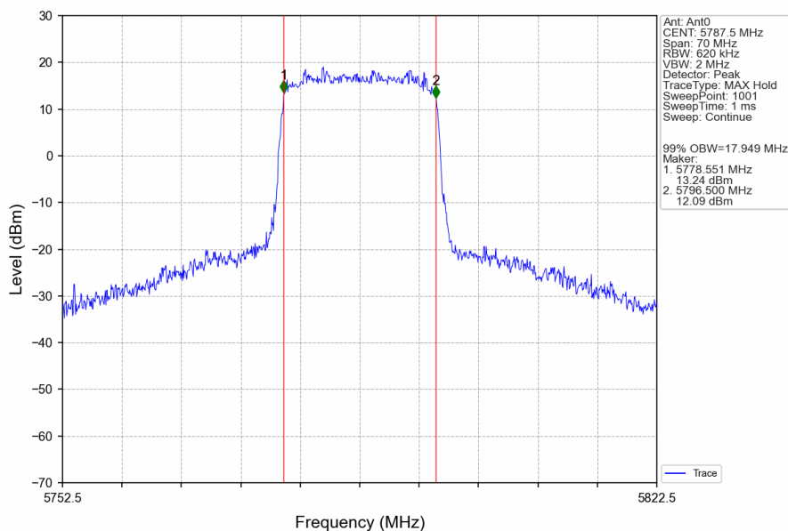
20M_MCH_5787.5MHz_Ant0_NTNV
