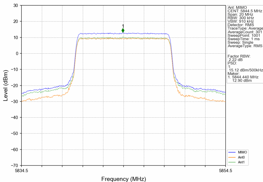
10M_HCH_5844.5MHz_MIMO_NTNV
