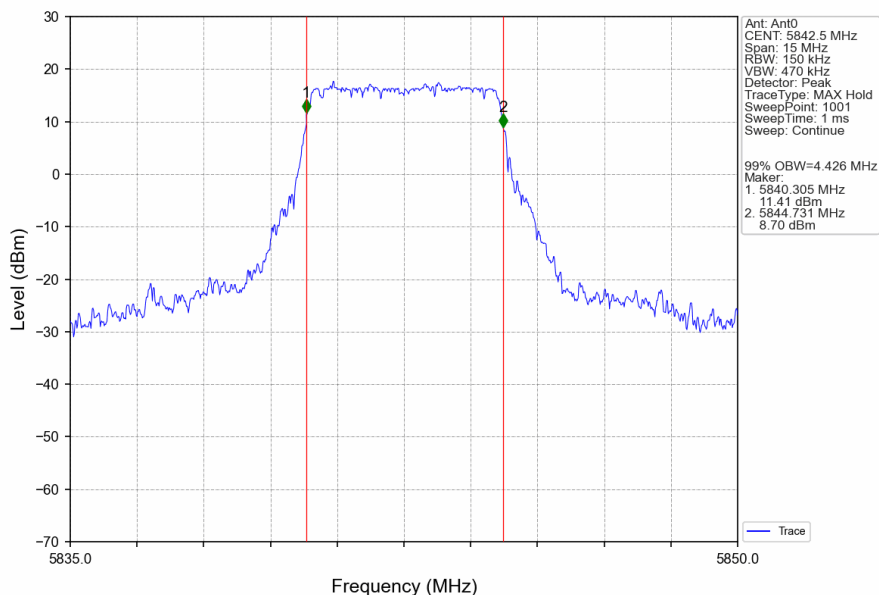
5M_HCH_5842.5MHz_Ant0_NTNV
