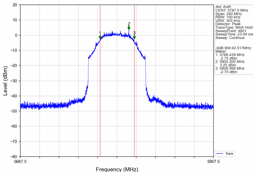
80M_MCH_5787.5MHz_Ant0_NTNV
