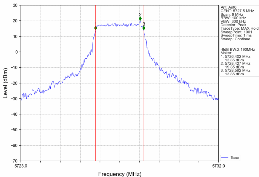
3M_LCH_5727.5MHz_Ant0_NTNV
