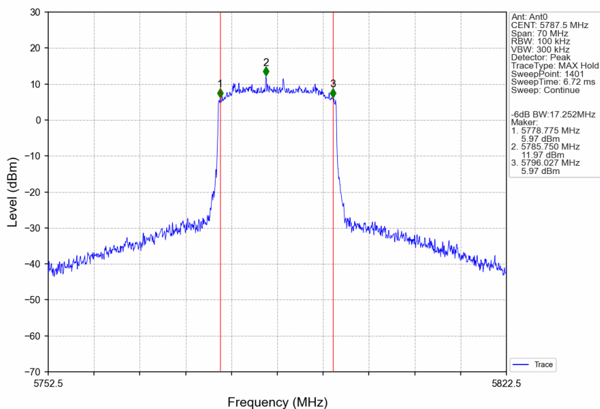
20M_MCH_5787.5MHz_Ant0_NTNV
