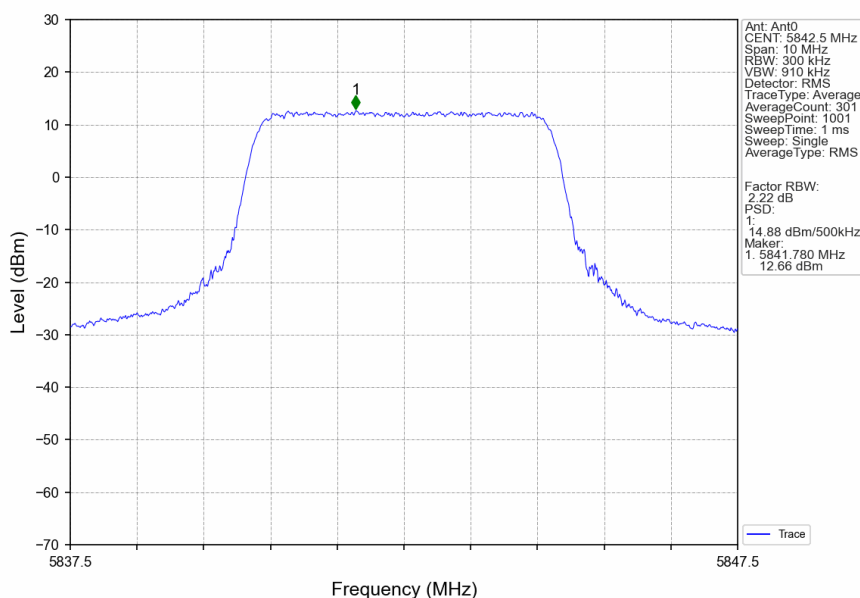
5M_HCH_5842.5MHz_Ant0_NTNV
