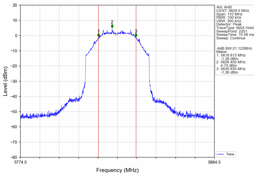
40M_HCH_5829.5MHz_Ant0_NTNV
