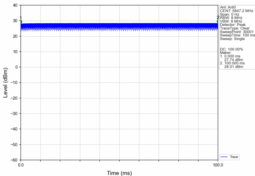
3M_HCH_5847.2MHz_Ant0_NTNV
