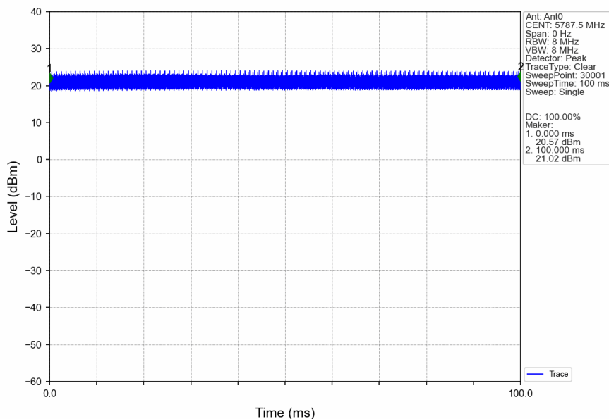
40M_MCH_5787.5MHz_Ant0_NTNV
