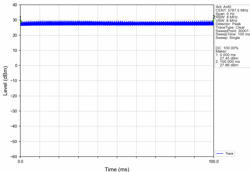
10M_MCH_5787.5MHz_Ant0_NTNV
