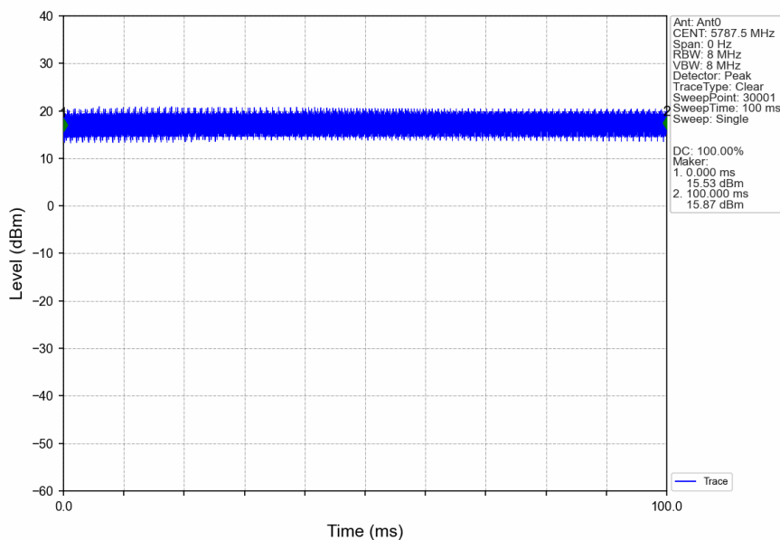
60M_MCH_5787.5MHz_Ant0_NTNV
