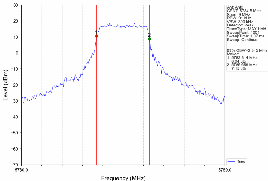
3M_MCH_5784.5MHz_Ant0_NTNV
