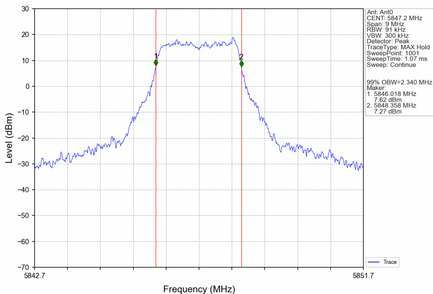
3M_HCH_5847.2MHz_Ant0_NTNV
