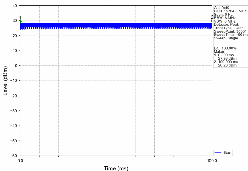
3M_MCH_5784.5MHz_Ant0_NTNV
