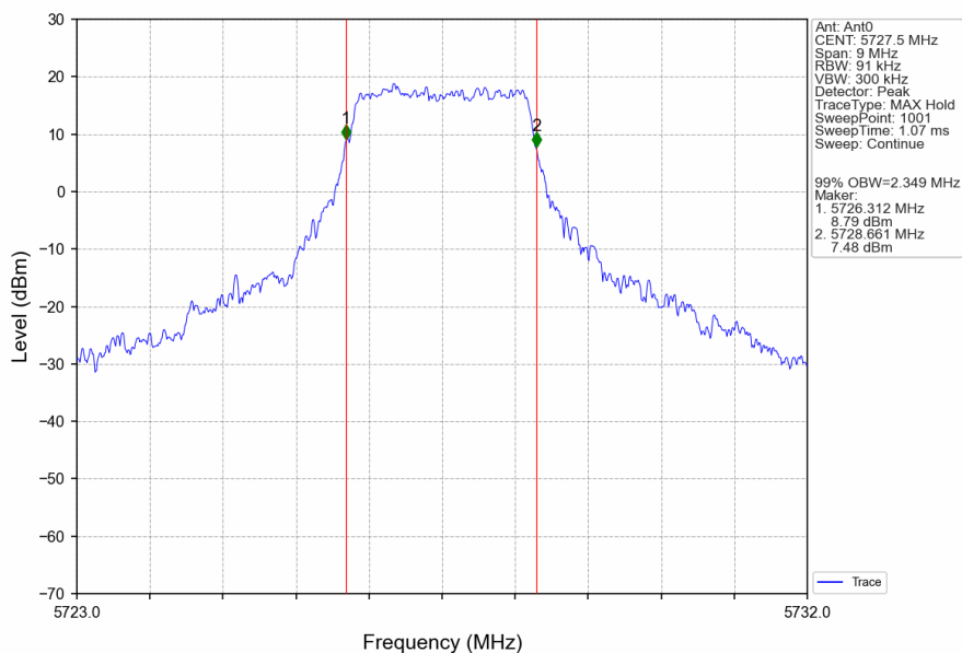
3M_LCH_5727.5MHz_Ant0_NTNV
