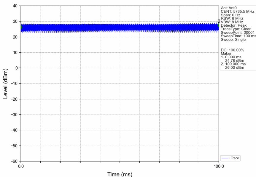
20M_LCH_5735.5MHz_Ant0_NTNV
