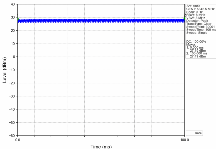
5M_HCH_5842.5MHz_Ant0_NTNV
