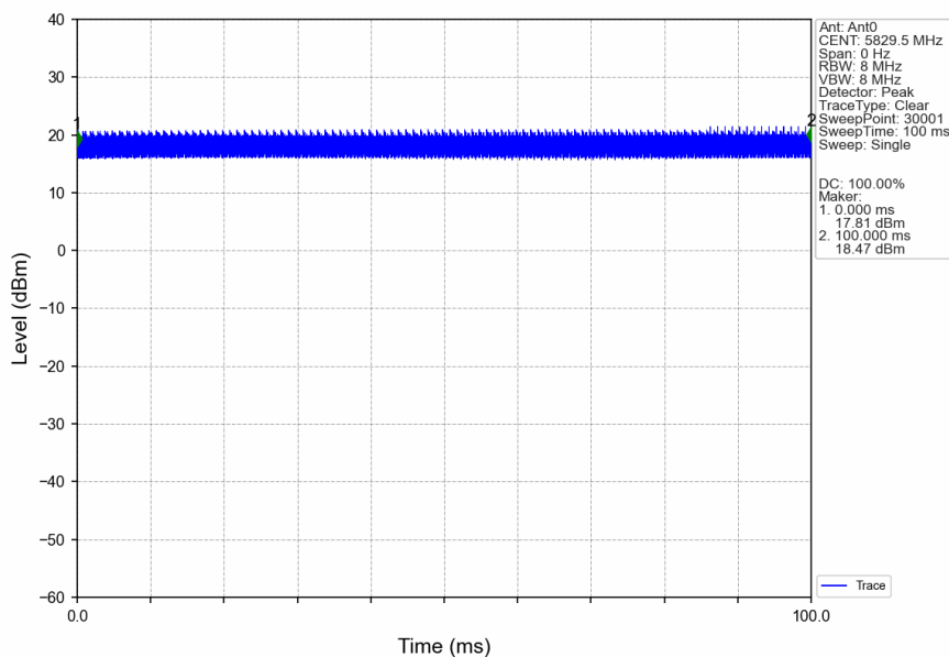
40M_HCH_5829.5MHz_Ant0_NTNV
