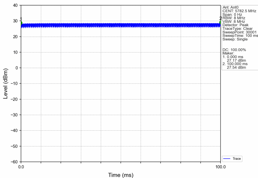
5M_MCH_5782.5MHz_Ant0_NTNV
