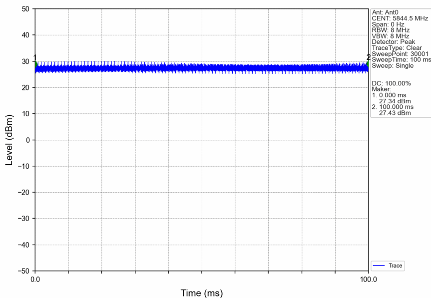
10M_HCH_5844.5MHz_Ant0_NTNV
