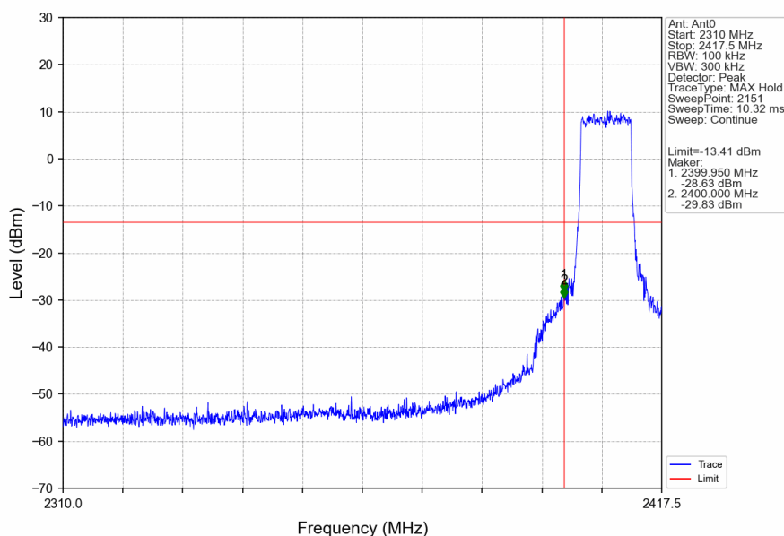
10M_LCH_2407.5MHz_Ant0_NTNV
