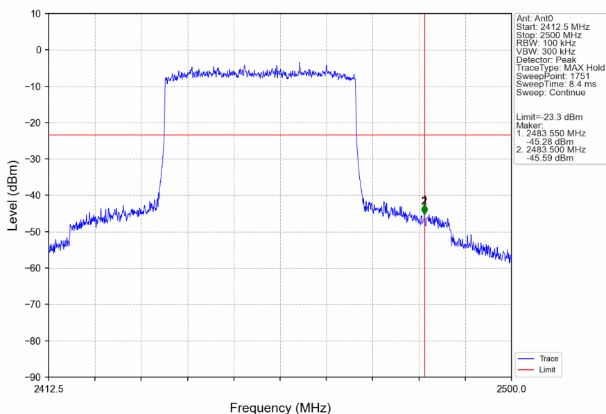
40M_HCH_2452.5MHz_Ant0_NTNV
