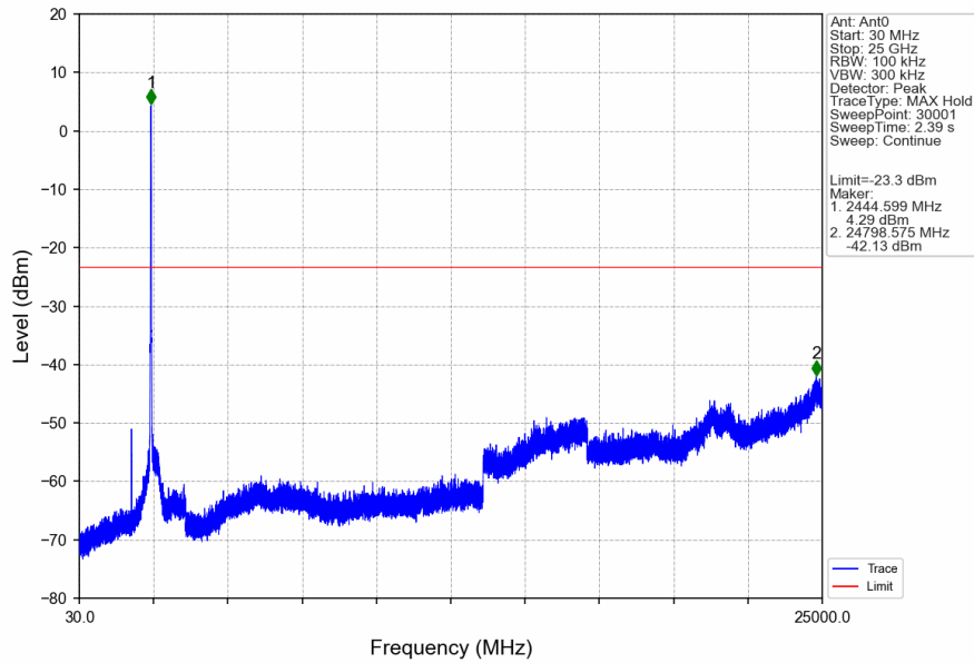
40M_MCH_2437.5MHz_Ant0_NTNV
