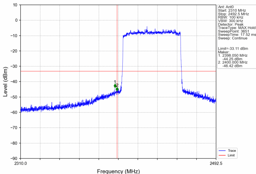
60M_LCH_2432.5MHz_Ant0_NTNV
