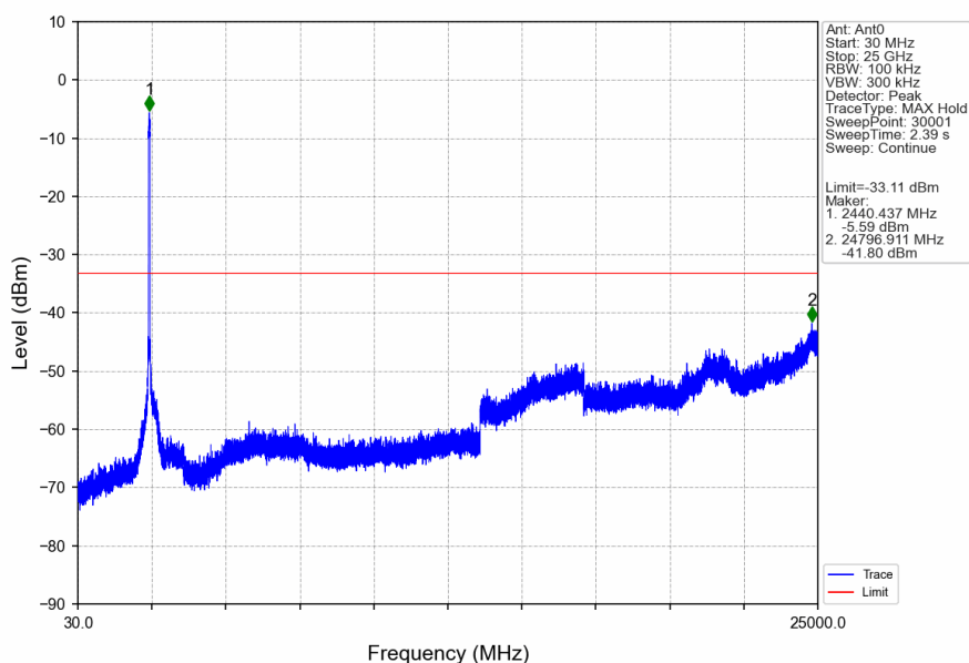
60M_MCH_2437.5MHz_Ant0_NTNV
