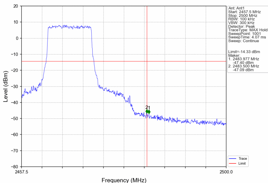
10M_HCH_2467.5MHz_Ant1_NTNV
