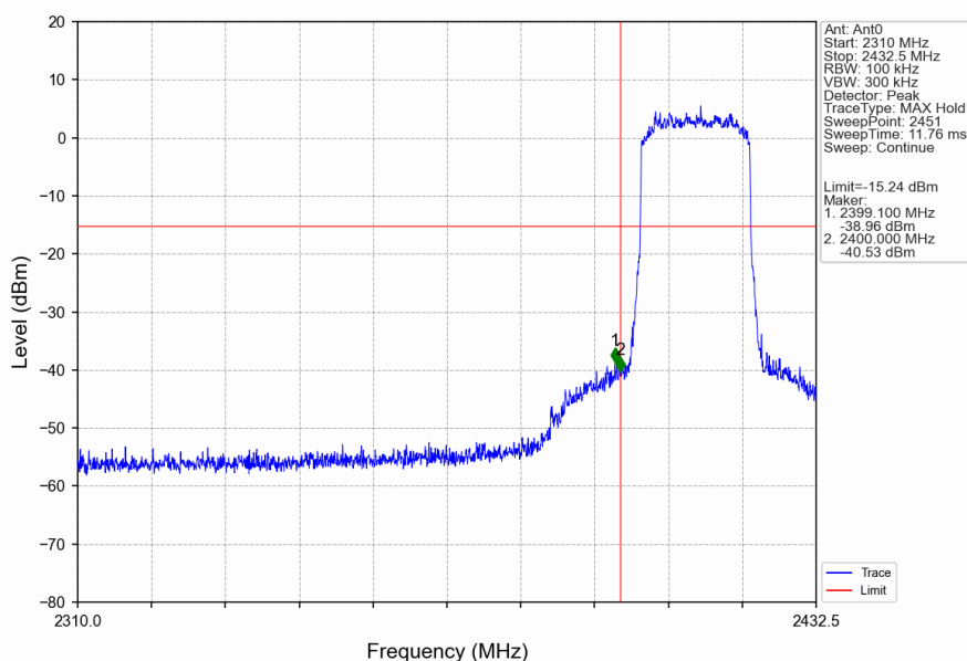
20M_LCH_2412.5MHz_Ant0_NTNV
