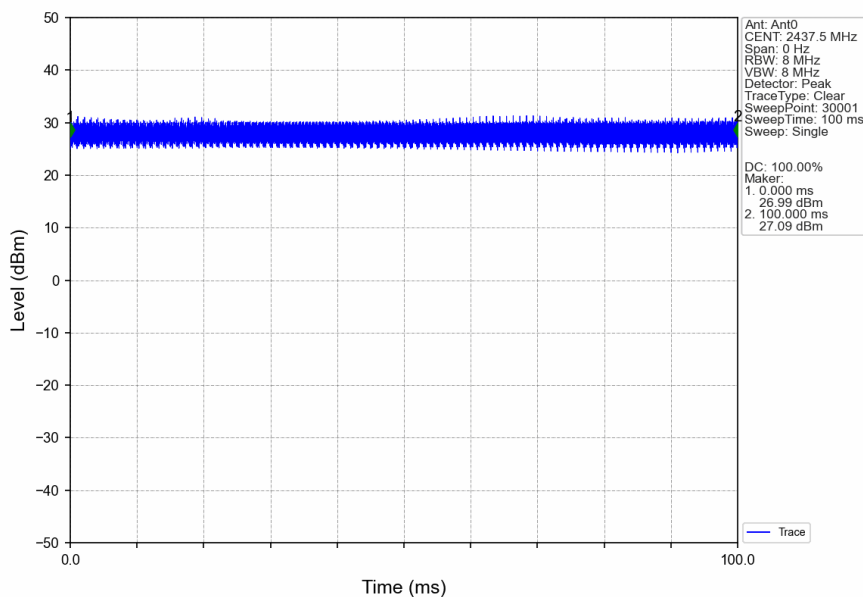
20M_MCH_2437.5MHz_Ant0_NTNV
