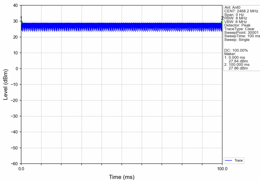
3M_HCH_2468.2MHz_Ant0_NTNV
