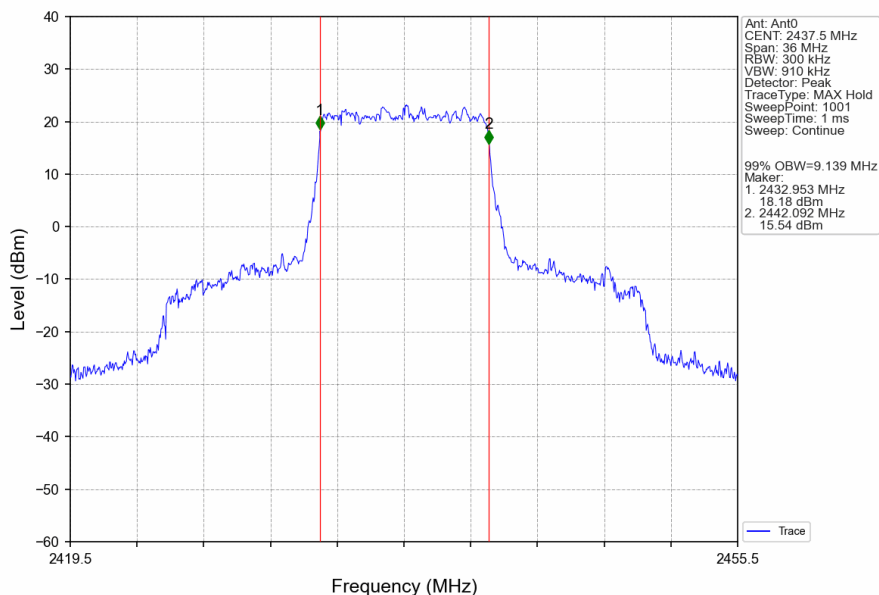
10M_MCH_2437.5MHz_Ant0_NTNV
