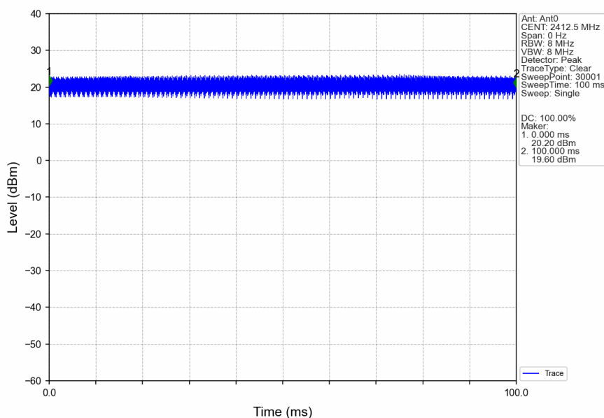
20M_LCH_2412.5MHz_Ant0_NTNV
