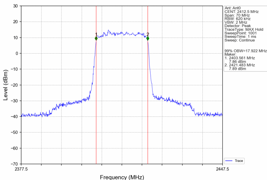
20M_LCH_2412.5MHz_Ant0_NTNV
