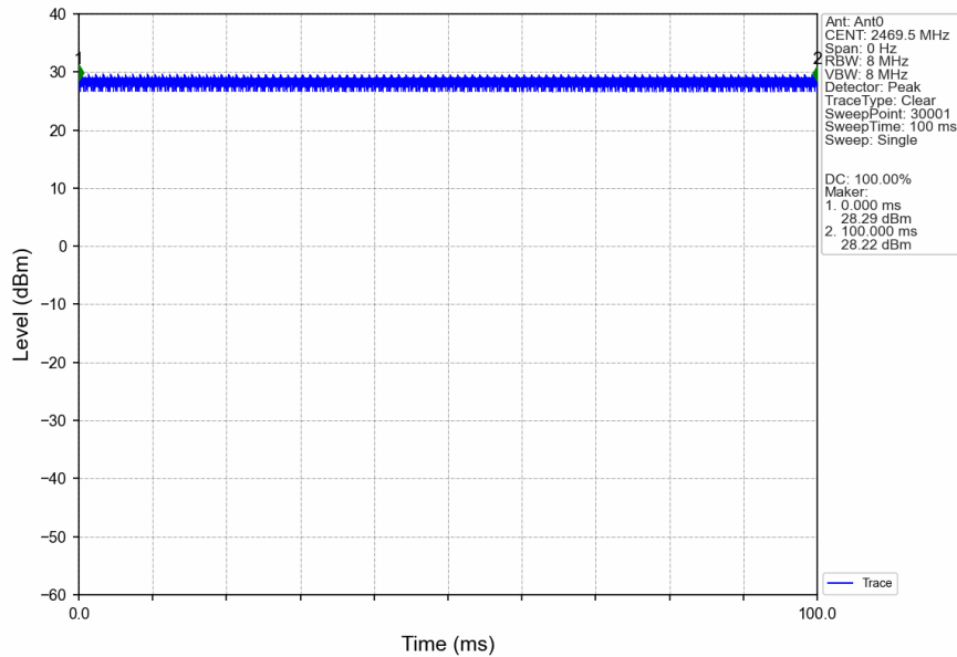
5M_HCH_2469.5MHz_Ant0_NTNV
