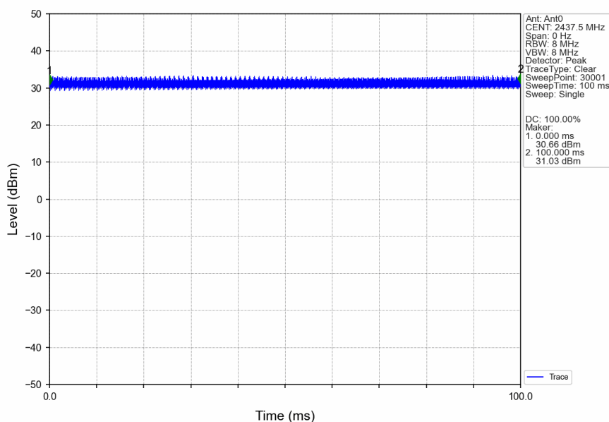
10M_MCH_2437.5MHz_Ant0_NTNV
