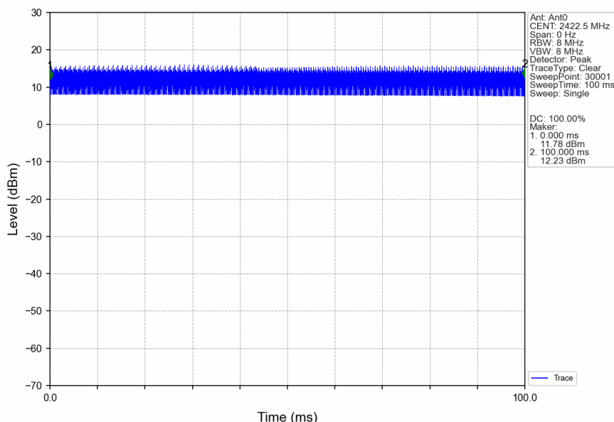
40M_LCH_2422.5MHz_Ant0_NTNV
