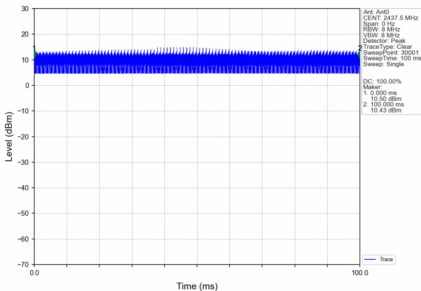
60M_MCH_2437.5MHz_Ant0_NTNV
