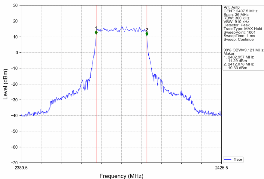
10M_LCH_2407.5MHz_Ant0_NTNV
