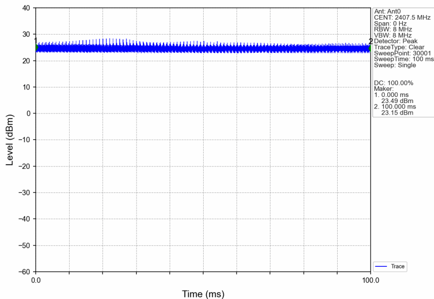
10M_LCH_2407.5MHz_Ant0_NTNV
