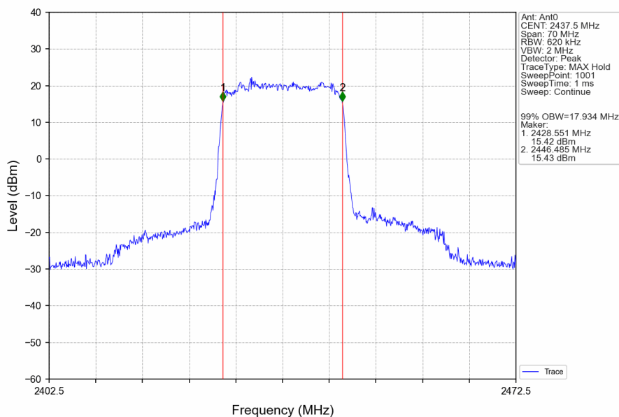
20M_MCH_2437.5MHz_Ant0_NTNV
