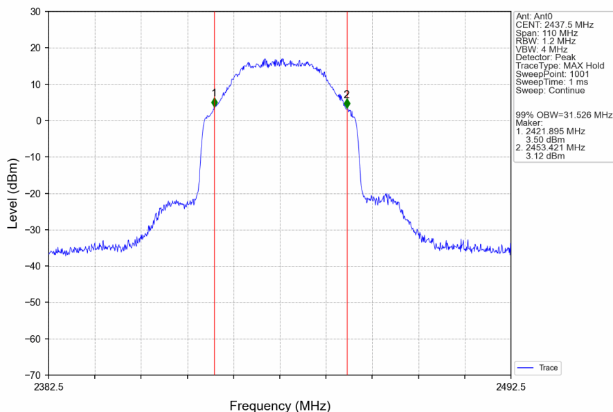
40M_MCH_2437.5MHz_Ant0_NTNV
