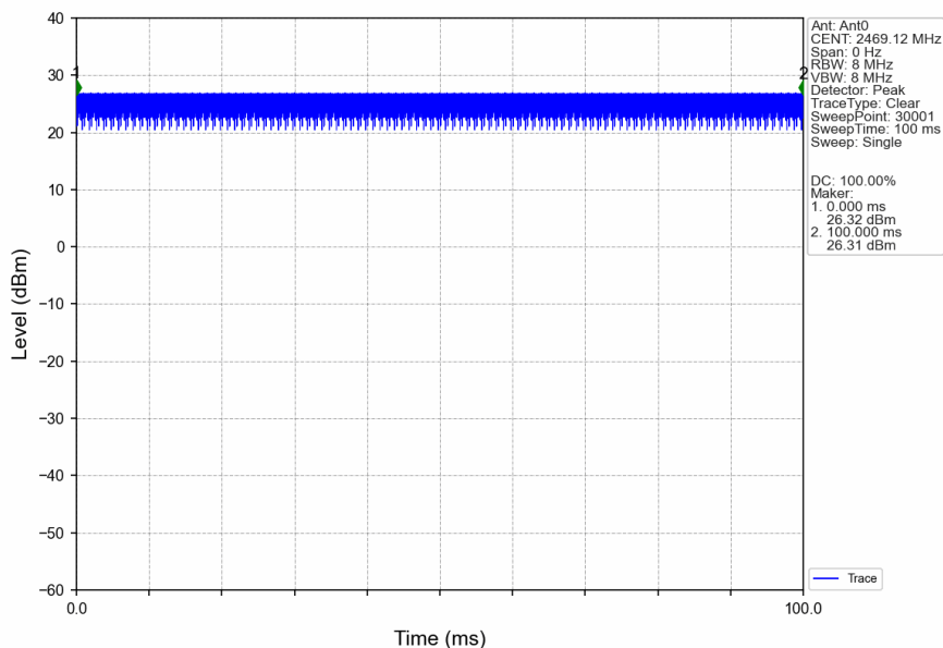
1.4M_HCH_2469.12MHz_Ant0_NTNV
