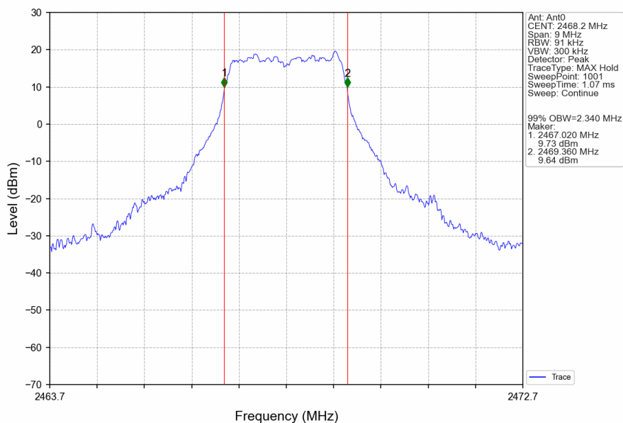
3M_HCH_2468.2MHz_Ant0_NTNV
