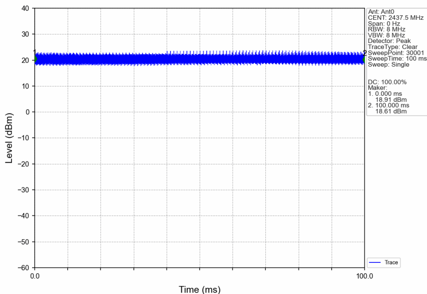
40M_MCH_2437.5MHz_Ant0_NTNV
