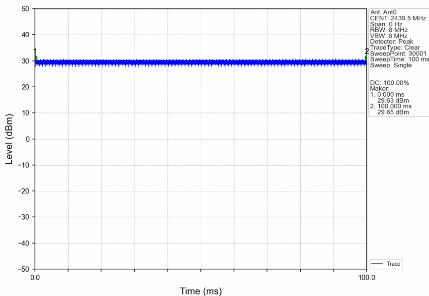
5M_MCH_2439.5MHz_Ant0_NTNV
