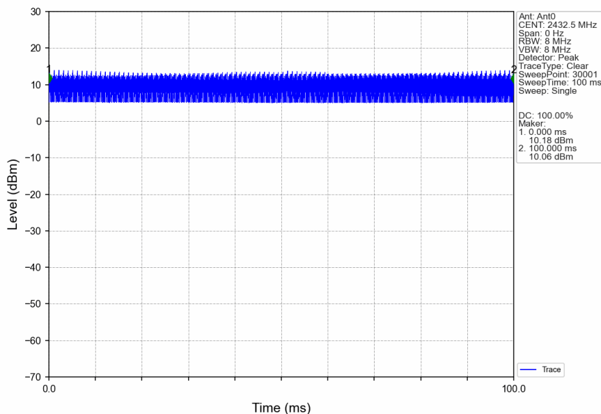
60M_LCH_2432.5MHz_Ant0_NTNV
