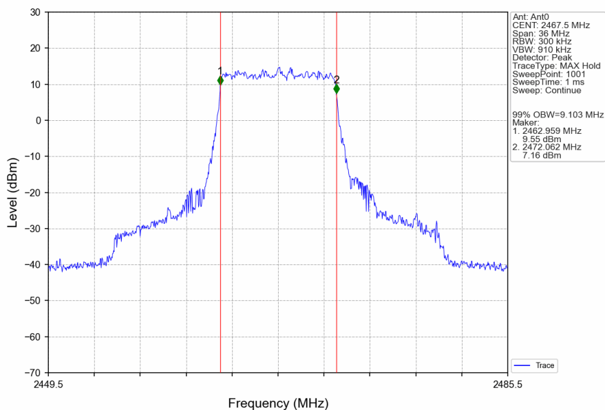
10M_HCH_2467.5MHz_Ant0_NTNV
