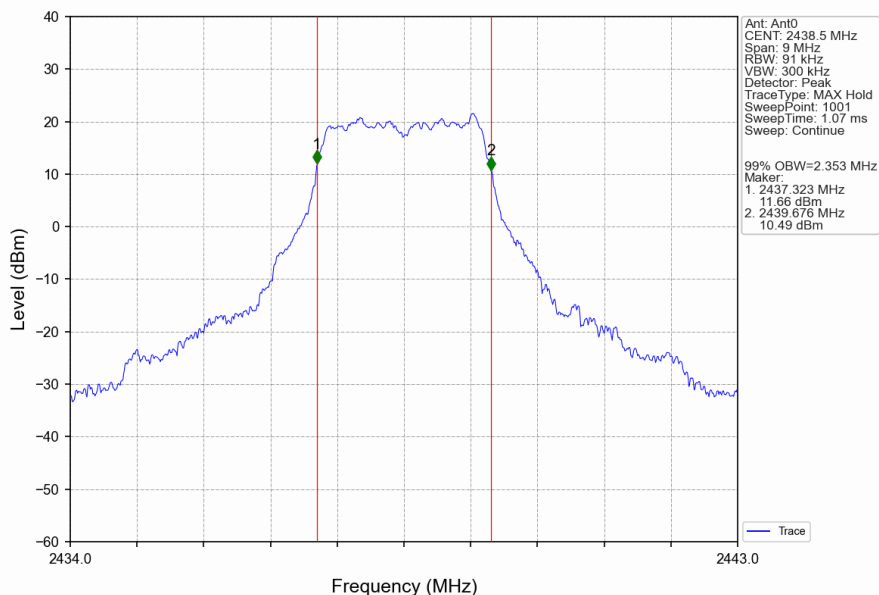
3M_MCH_2438.5MHz_Ant0_NTNV
