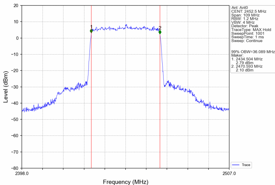
40M_HCH_2452.5MHz_Ant0_NTNV
