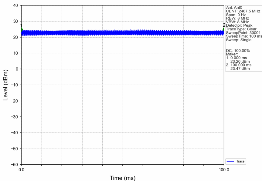
10M_HCH_2467.5MHz_Ant0_NTNV
