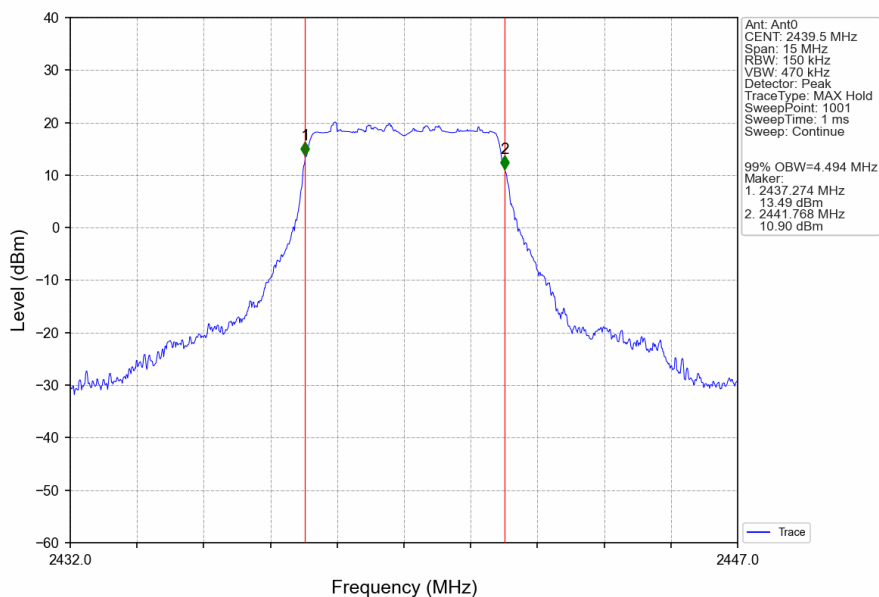
5M_MCH_2439.5MHz_Ant0_NTNV
