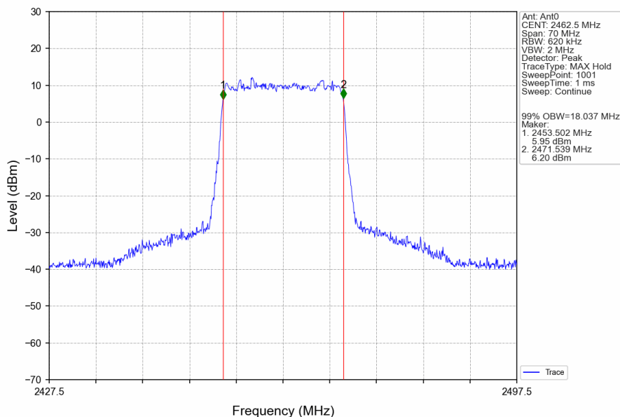
20M_HCH_2462.5MHz_Ant0_NTNV
