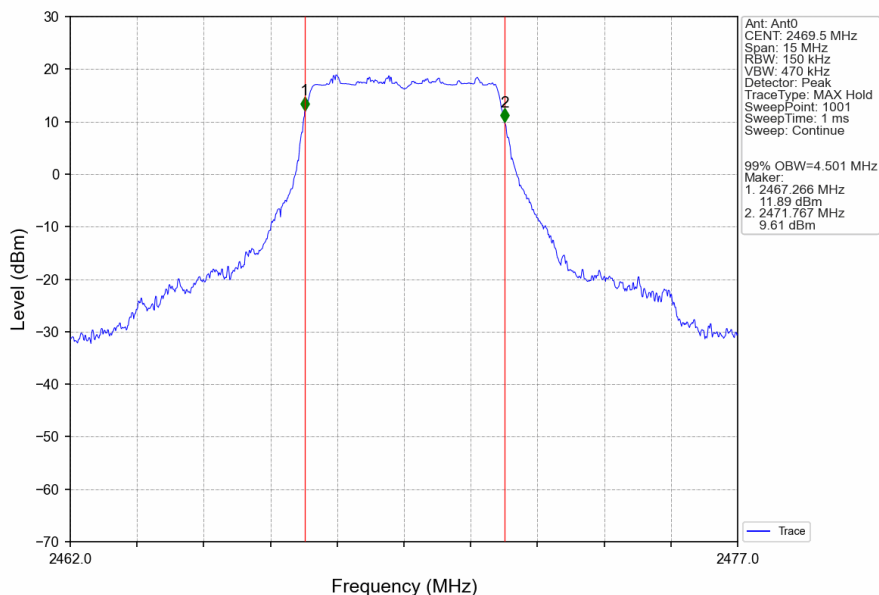
5M_HCH_2469.5MHz_Ant0_NTNV
