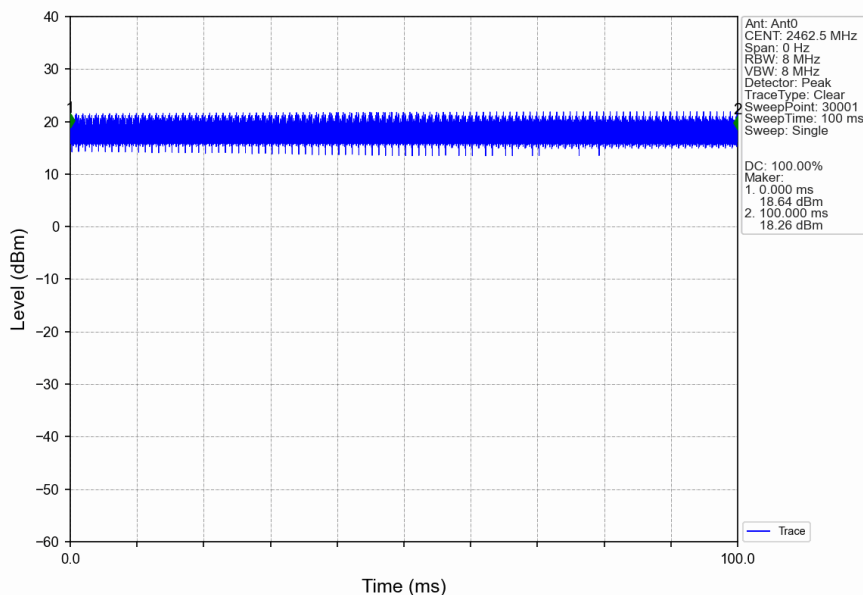
20M_HCH_2462.5MHz_Ant0_NTNV
