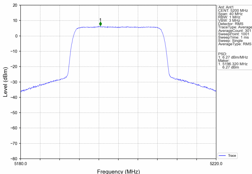
20M_MCH_5200MHz_Ant1_NTNV
