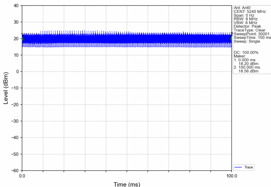
20M_HCH_5240MHz_Ant0_NTNV
