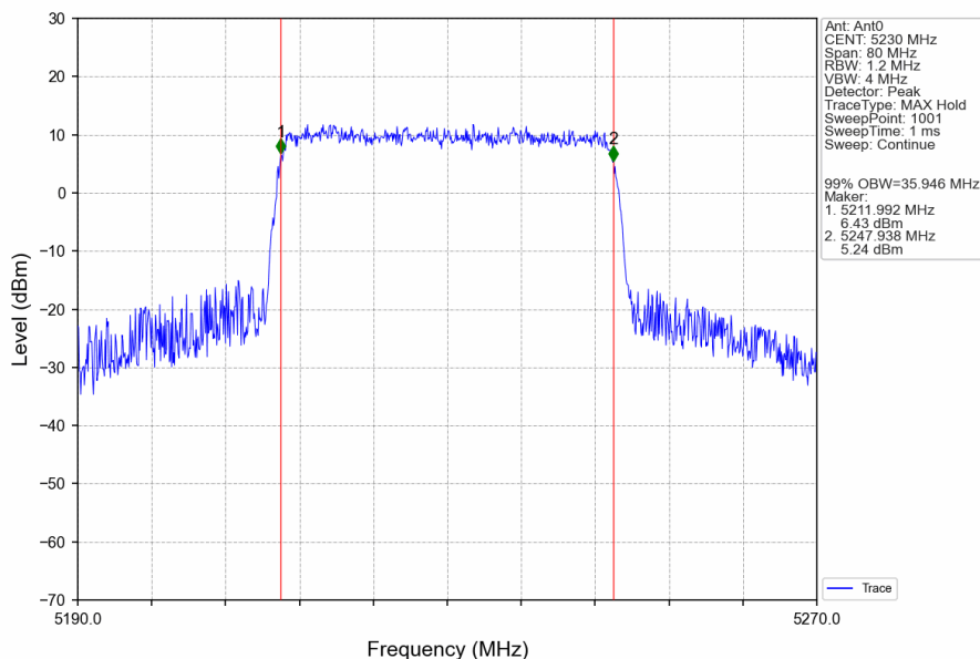
40M_HCH_5230MHz_Ant0_NTNV
