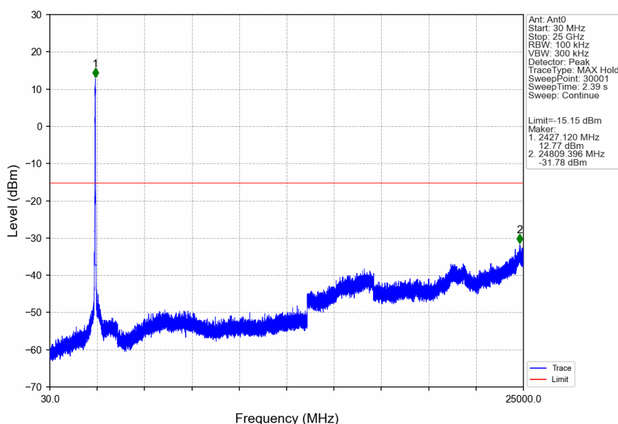
40M_LCH_2422.5MHz_Ant0_NTNV
