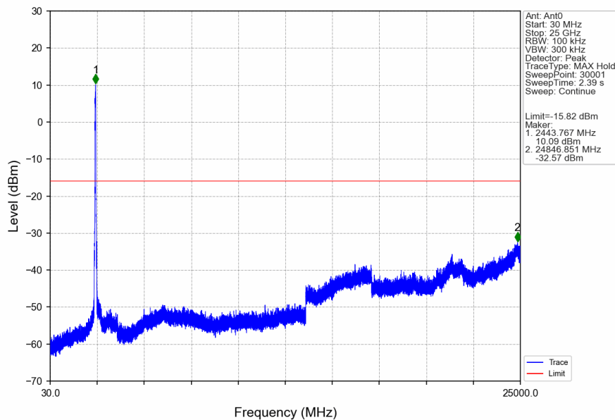
60M_LCH_2432.5MHz_Ant0_NTNV
