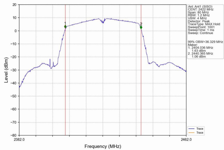
802.11n(HT40)_LCH_2422MHz_Ant1 (SISO)_NTNV
