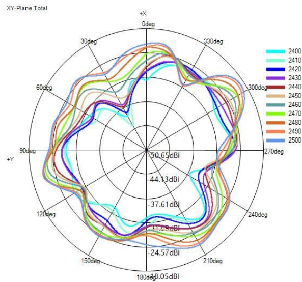
(3)X-Y Plane(unit:dBi):
