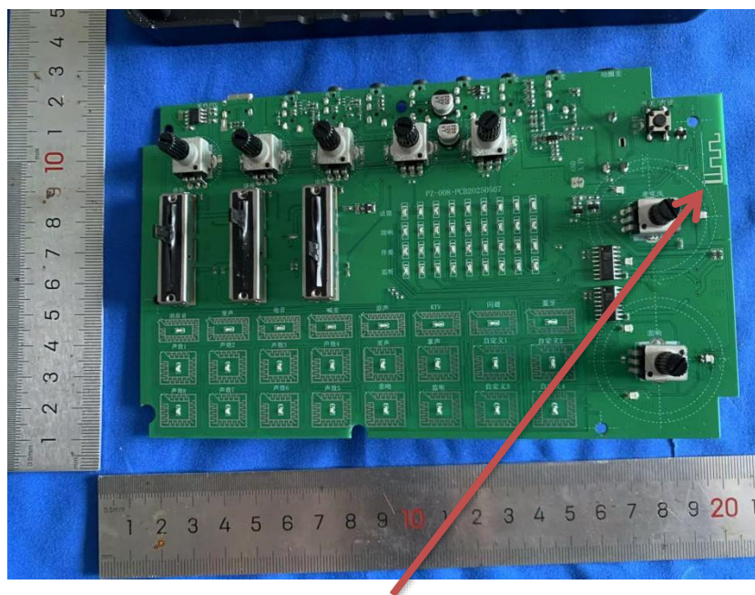
Antenna
