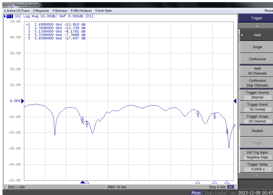
Main天线S11
