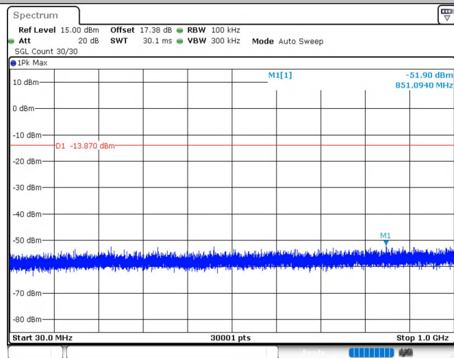
11B_Ant1_2437_0~Reference
