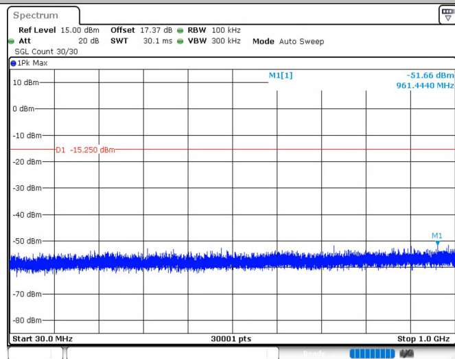
11B_Ant1_2462_0~Reference
