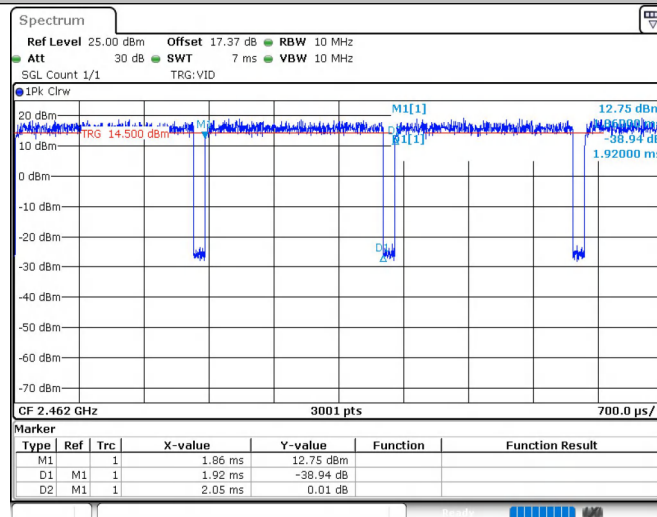
11N20SISO_Ant1_2462
