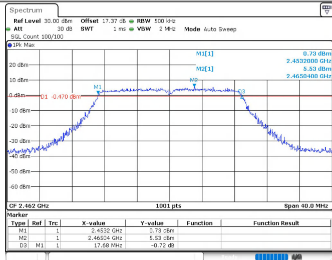
11N20SISO_Ant1_2462
