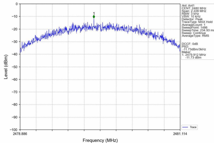
2M_HCH_2480MHz_Ant1_NTNV
