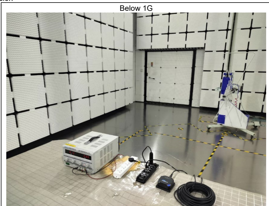
9kHz-30MHz
