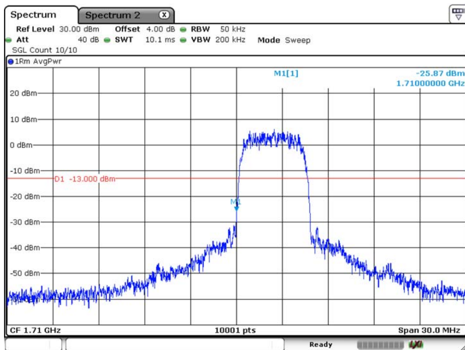
WCDMA_Band 4_RMC_1712.4
