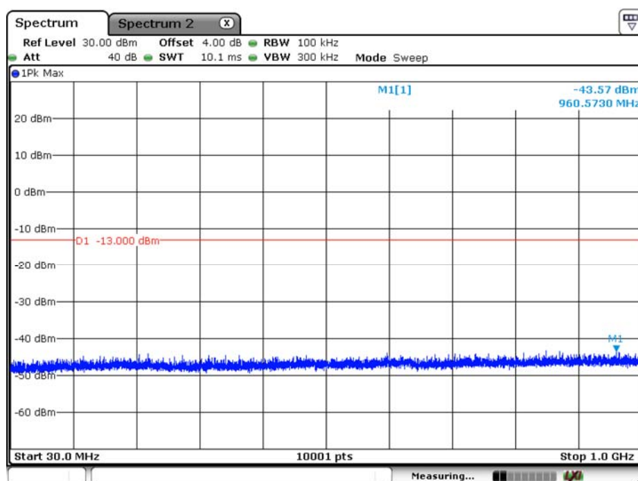
WCDMA_B2_CH9262_RMC_under 1G
