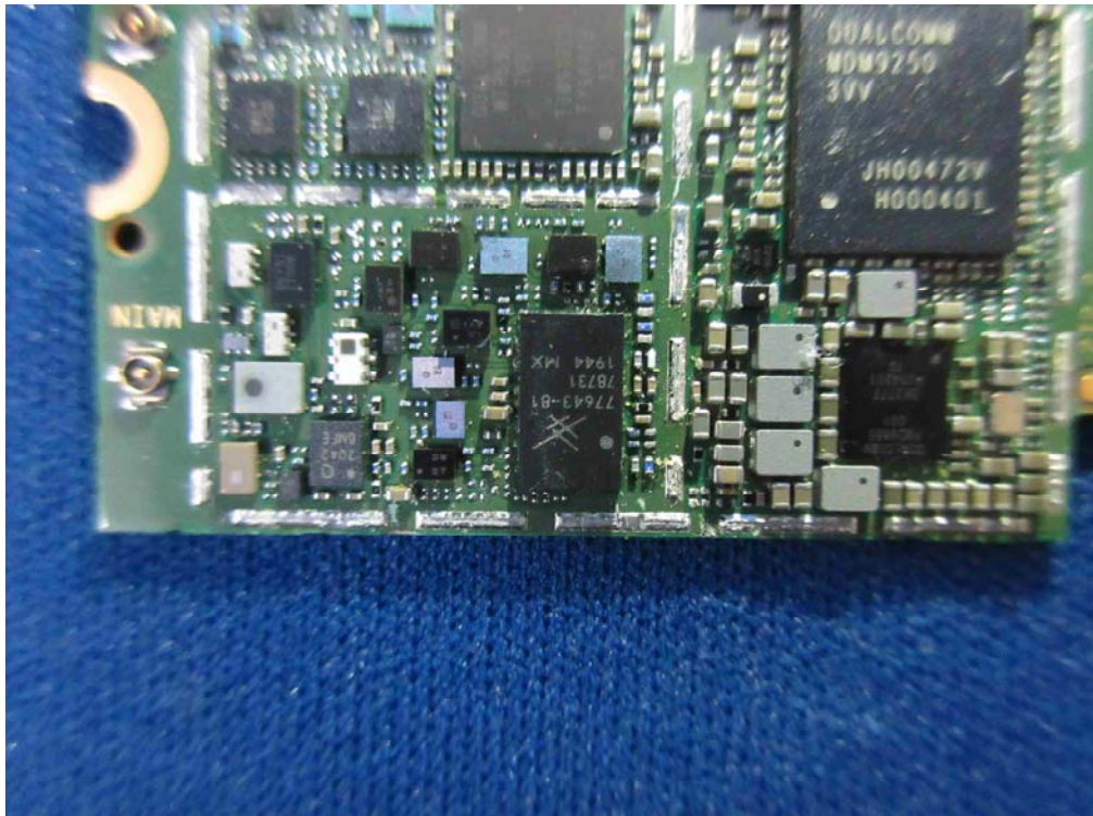
(18) EUT Photo
