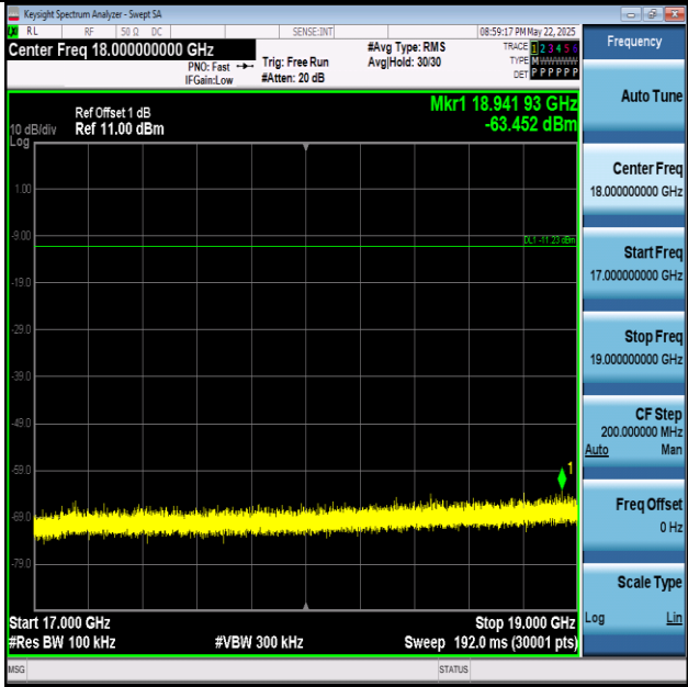
BLE_2M-Ant1-2440-17000~19000-PASS
