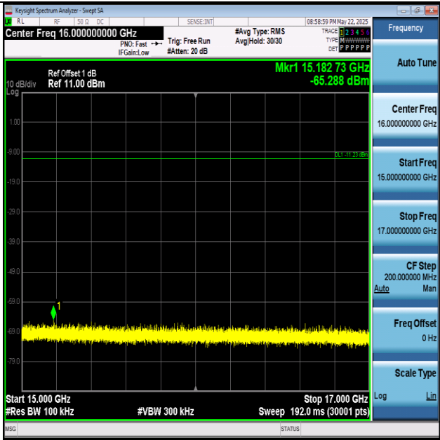
BLE_2M-Ant1-2440-15000~17000-PASS
