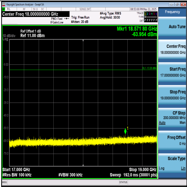
BLE_2M-Ant1-2402-17000~19000-PASS
