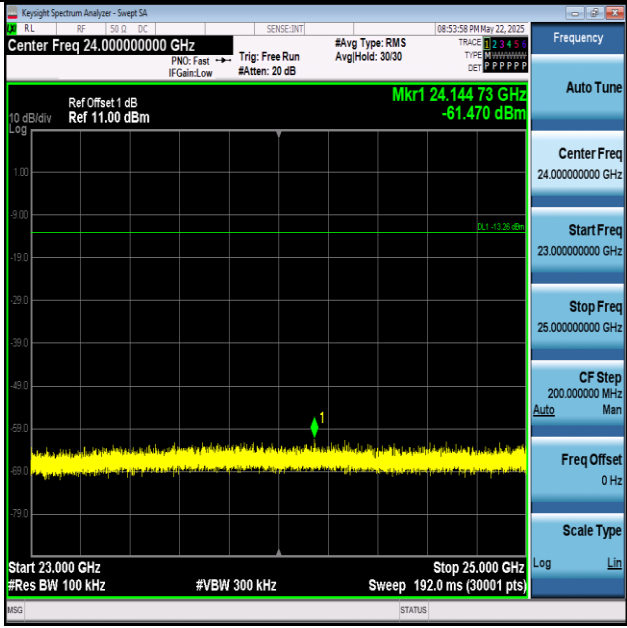
BLE_2M-Ant1-2402-23000~25000-PASS
