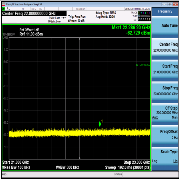
BLE_2M-Ant1-2402-21000~23000-PASS
