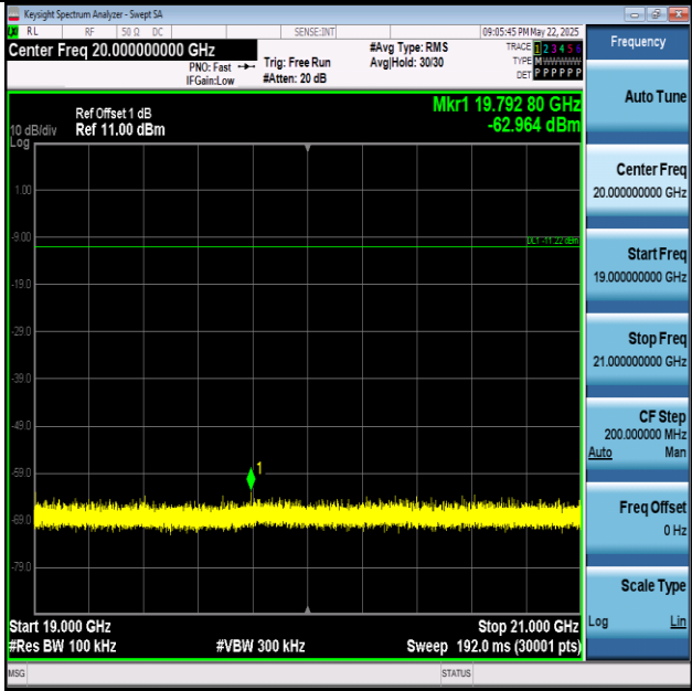
BLE_2M-Ant1-2480-19000~21000-PASS
