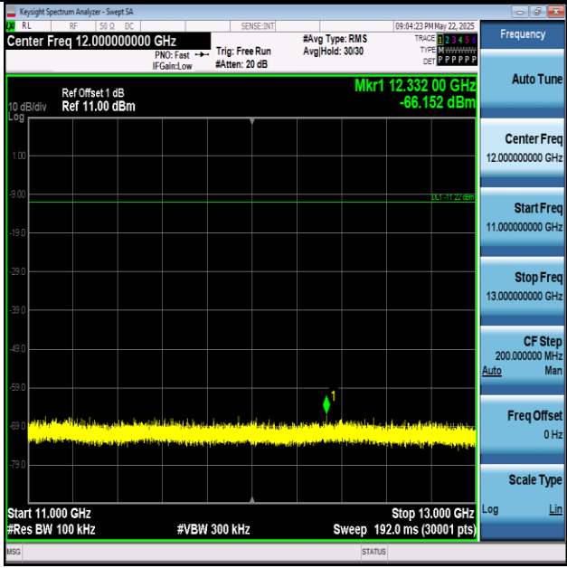
BLE_2M-Ant1-2480-11000~13000-PASS
