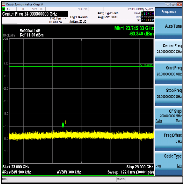
BLE_2M-Ant1-2440-23000~25000-PASS
