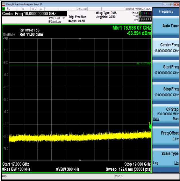
BLE_2M-Ant1-2480-17000~19000-PASS
