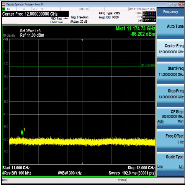
BLE_2M-Ant1-2440-11000~13000-PASS
