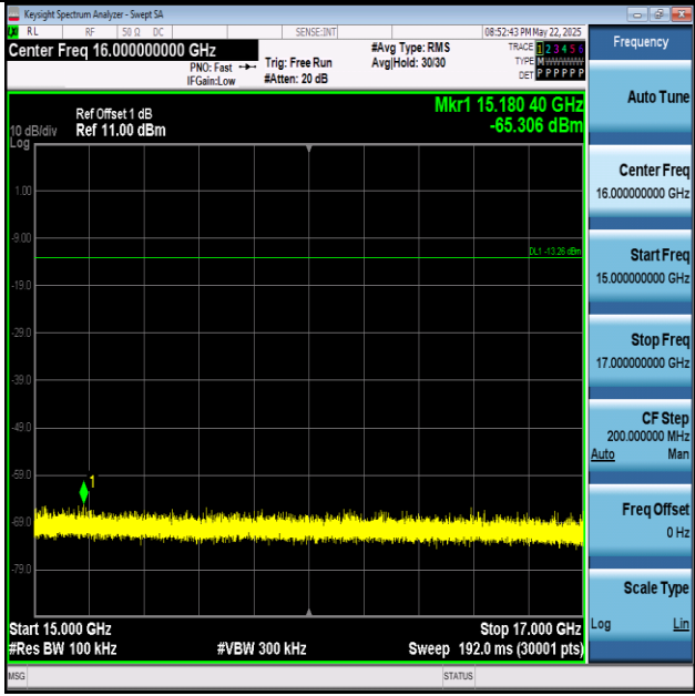
BLE_2M-Ant1-2402-15000~17000-PASS
