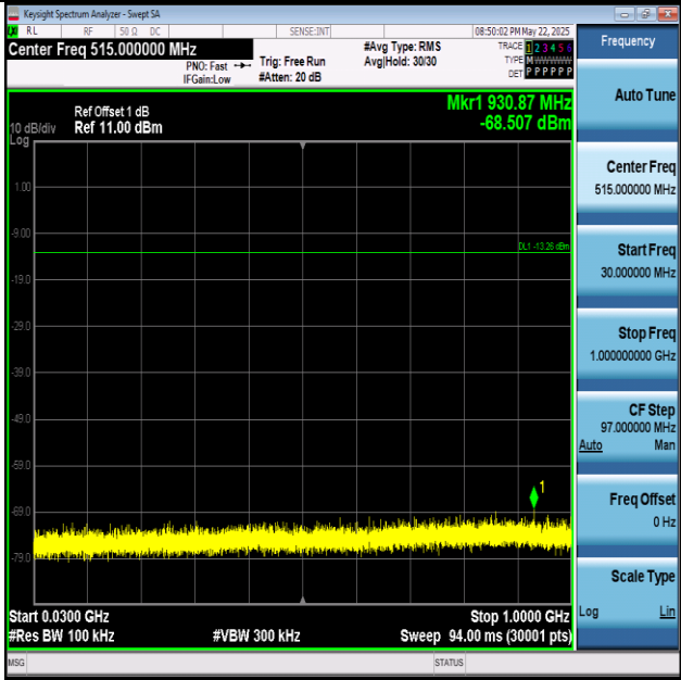
BLE_2M-Ant1-2402-30~1000-PASS
