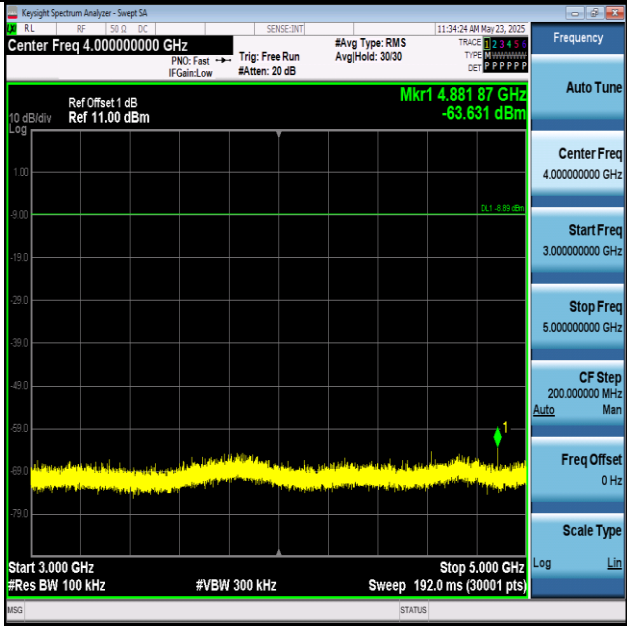
DH5-Ant1-2441-3000~5000-PASS
