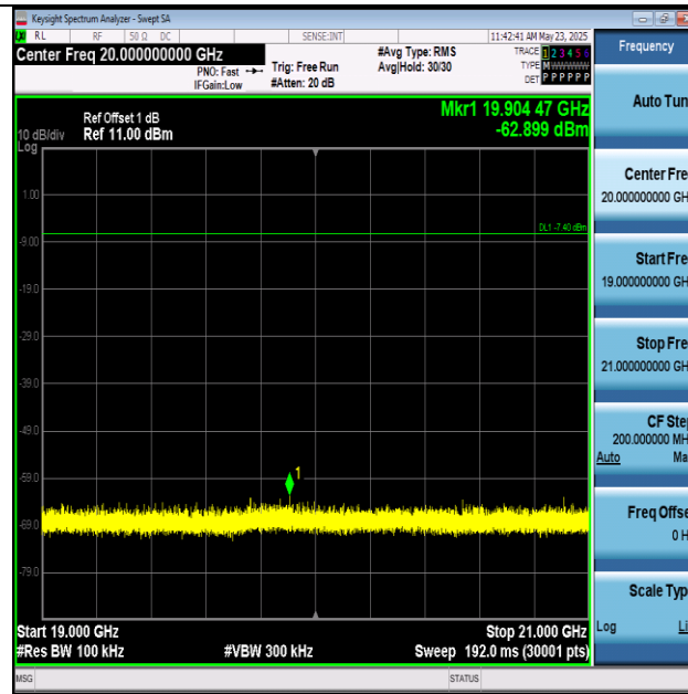
DH5-Ant1-2480-19000~21000-PASS
