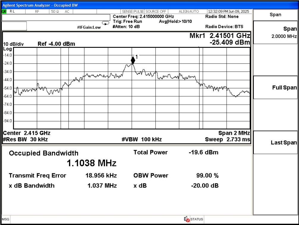
2415MHz
