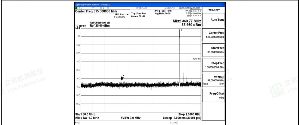
Band26-10MHz-16QAM-26840-1-0-Low-30-1000--37.56-PASS
