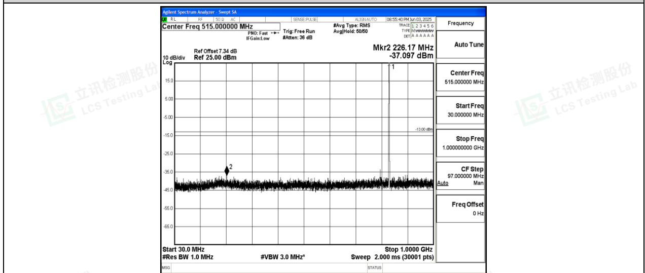
Band26-10MHz-QPSK-26915-1-0-Low-30-1000--37.1-PASS
