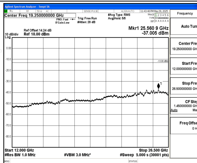
Band26-3MHz-16QAM-26740-1-0-Low-12000-26500--37.01-PASS
