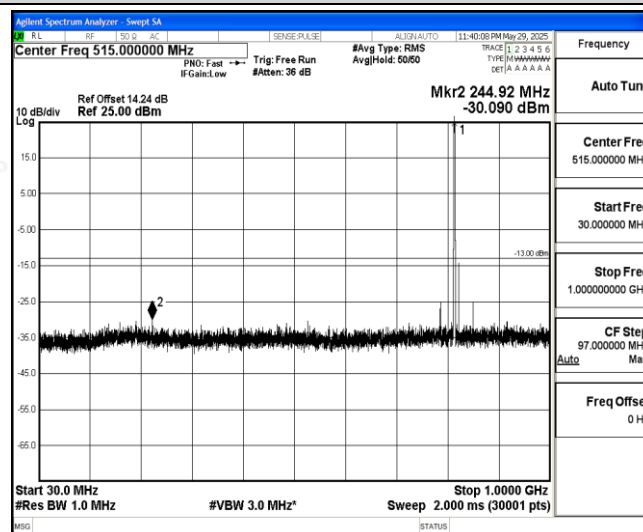
Band26-3MHz-QPSK-26740-1-0-Low-30-1000--30.09-PASS
