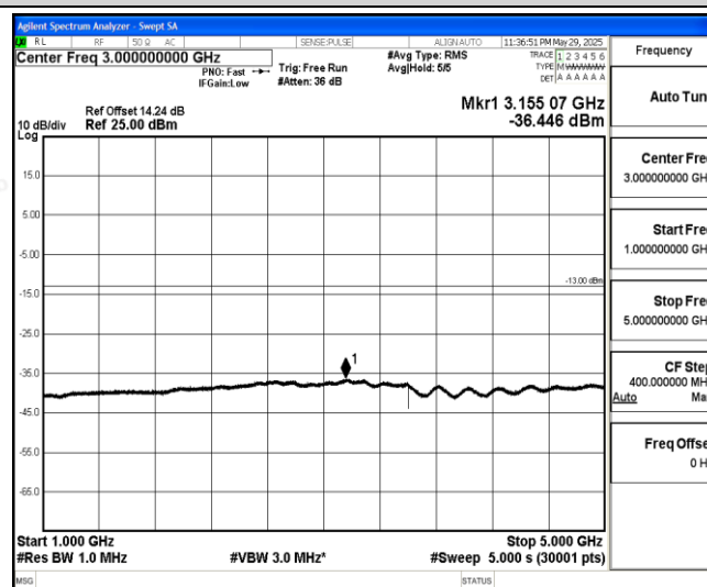
Band26-3MHz-QPSK-26705-1-0-Low-1000-5000--36.45-PASS
