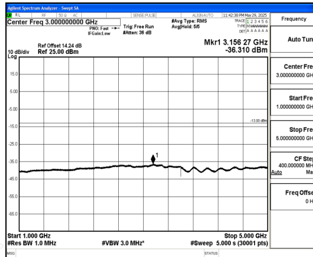
Band26-3MHz-16QAM-26740-1-0-Low-1000-5000--36.31-PASS
