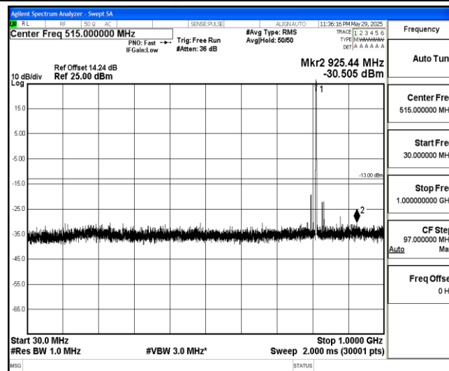
Band26-3MHz-QPSK-26705-1-0-Low-30-1000--30.51-PASS
