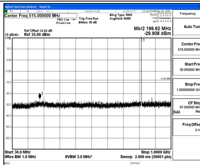
Band26-3MHz-16QAM-26740-1-0-Low-30-1000--29.91-PASS
