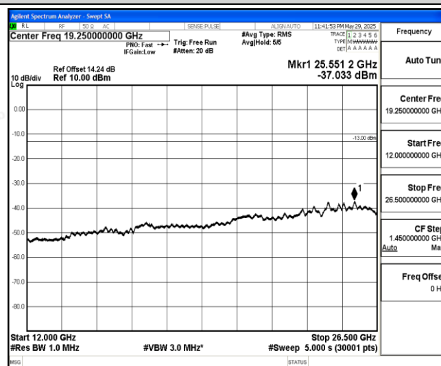
Band26-3MHz-QPSK-26740-1-0-Low-12000-26500--37.03-PASS
