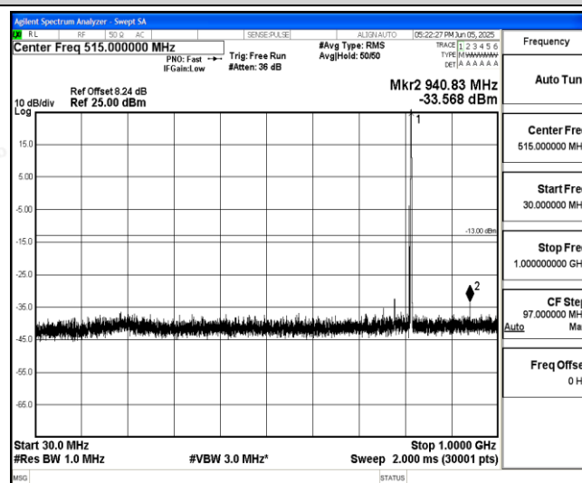
Band26-5MHz-QPSK-26740-1-0-Low-30-1000--33.57-PASS
