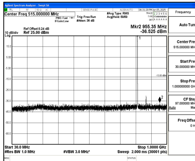
Band26-10MHz-QPSK-26740-1-0-Low-30-1000--36.53-PASS
