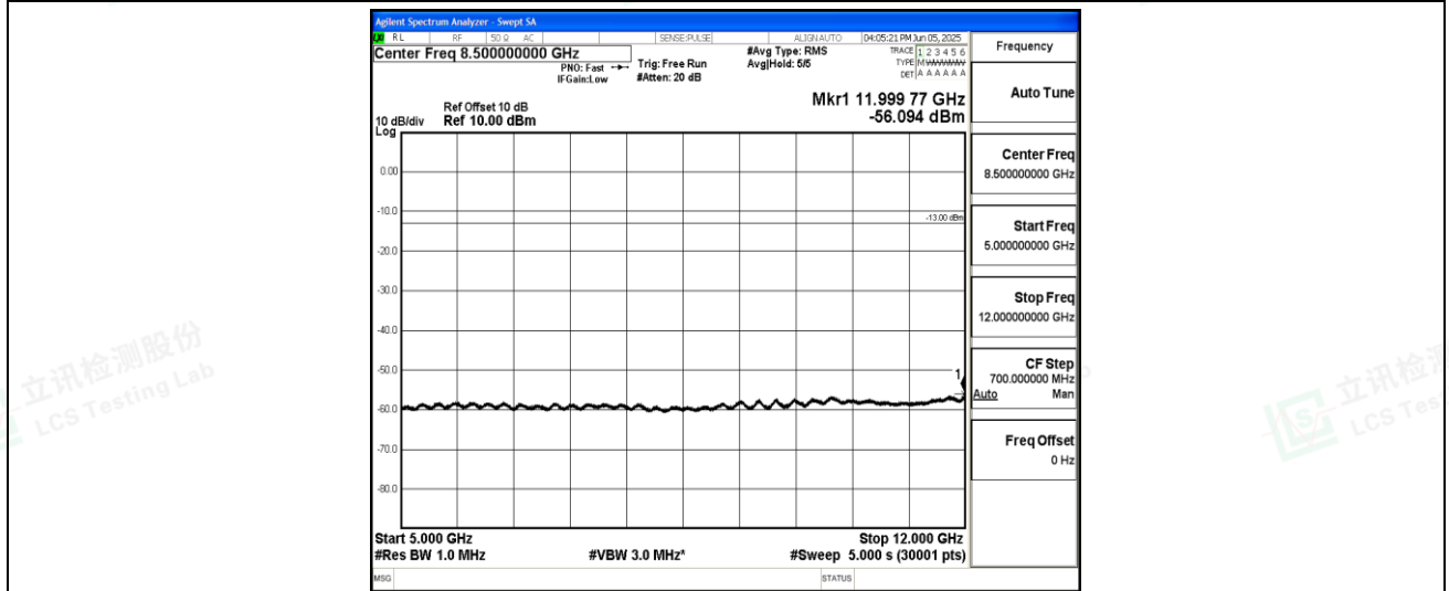
Band25-10MHz-QPSK-26365-1-0-Low-5000-12000--56.09-PASS
