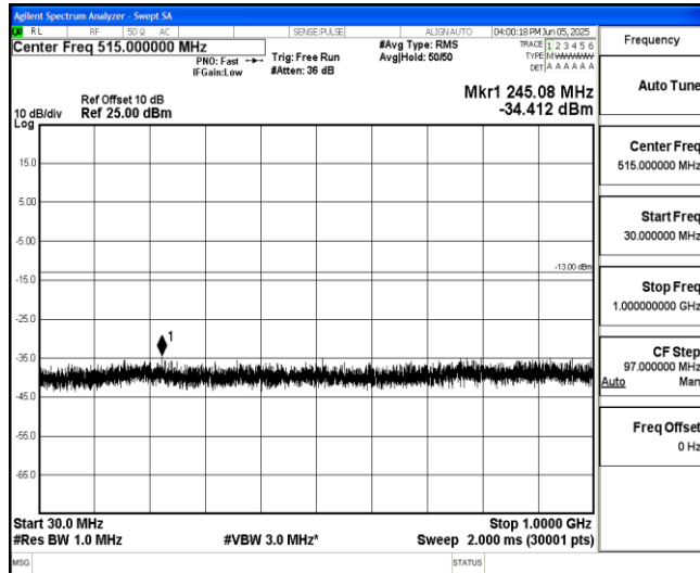
Band25-10MHz-QPSK-26090-1-0-Low-30-1000--34.41-PASS
