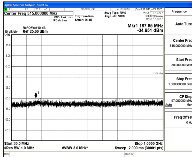
Band25-20MHz-16QAM-26140-1-0-Low-30-1000--34.85-PASS
