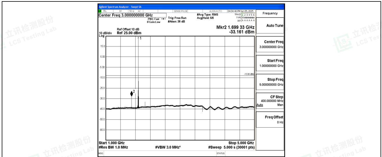
Band25-10MHz-QPSK-26365-1-0-Low-1000-5000--33.16-PASS
