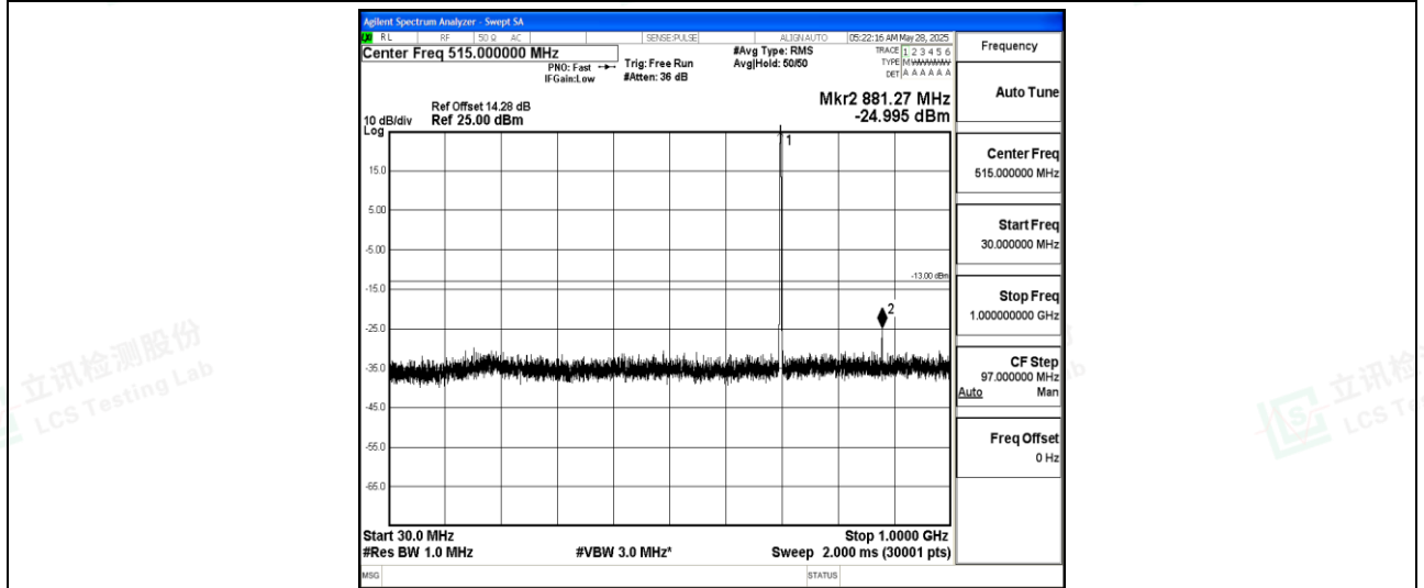
Band12-5MHz-QPSK-23095-1-0-Low-30-1000--25-PASS
