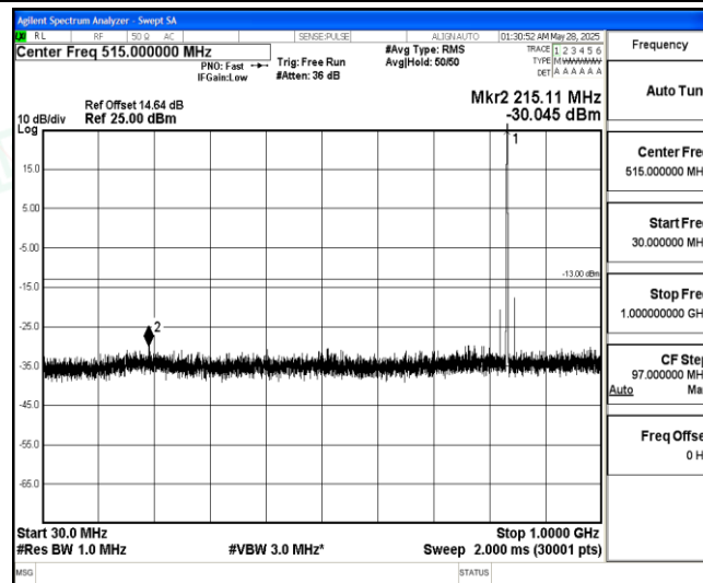
Band5-3MHz-QPSK-20525-1-0-Low-30-1000--30.05-PASS
