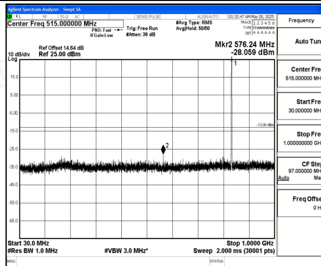
Band5-3MHz-16QAM-20525-1-0-Low-30-1000--28.06-PASS
