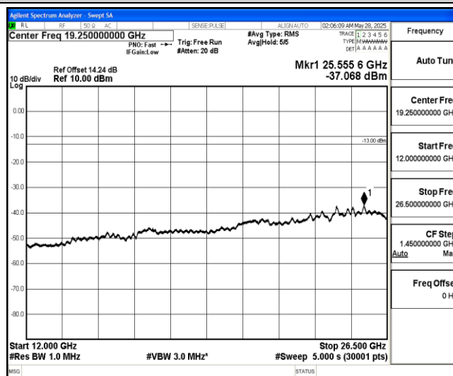
Band5-5MHz-QPSK-20425-1-0-Low-12000-26500--37.07-PASS
