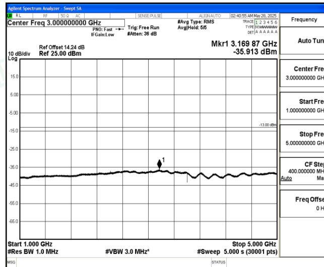
Band5-10MHz-QPSK-20450-1-0-Low-1000-5000--35.91-PASS
