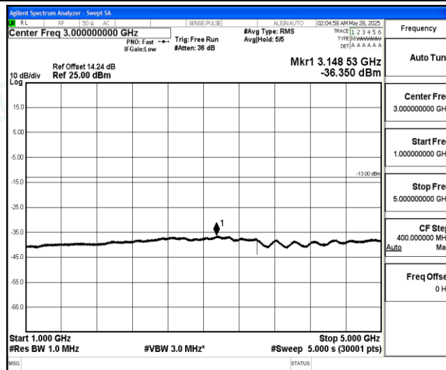
Band5-5MHz-QPSK-20425-1-0-Low-1000-5000--36.35-PASS
