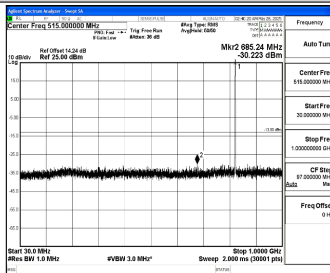
Band5-10MHz-QPSK-20450-1-0-Low-30-1000--30.22-PASS
