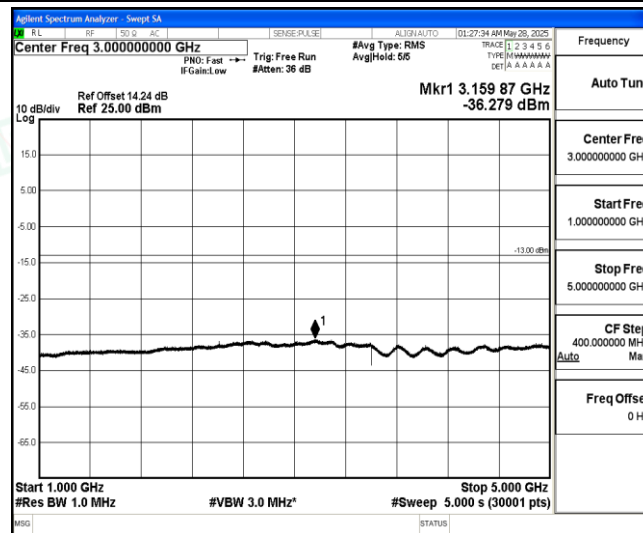
Band5-3MHz-QPSK-20415-1-0-Low-1000-5000--36.28-PASS
