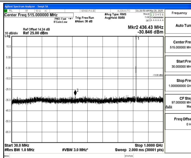
Band5-3MHz-QPSK-20415-1-0-Low-30-1000--30.85-PASS
