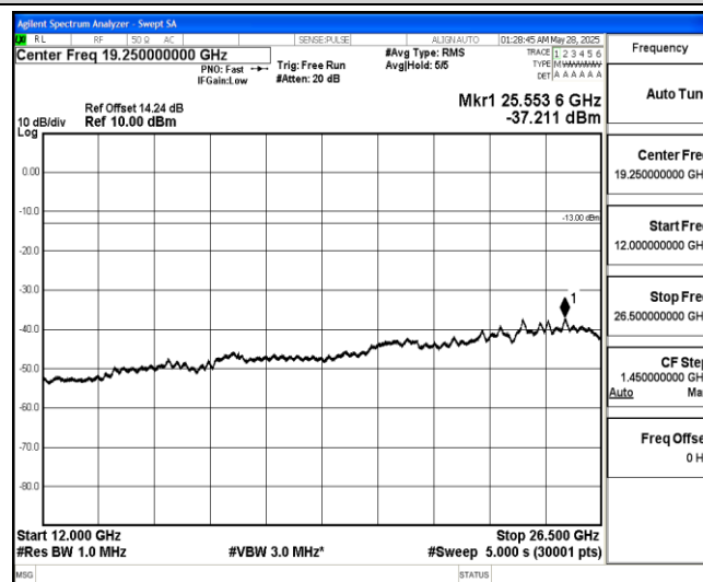
Band5-3MHz-QPSK-20415-1-0-Low-12000-26500--37.21-PASS
