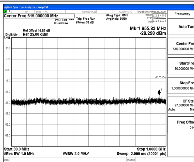
Band4-10MHz-16QAM-20000-1-0-Low-30-1000--28.3-PASS
