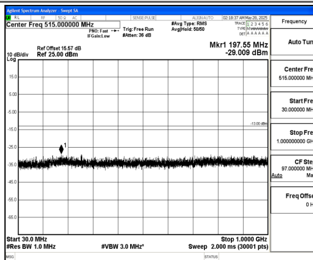
Band4-15MHz-QPSK-20025-1-0-Low-30-1000--29.01-PASS
