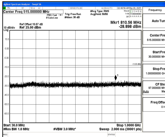
Band4-20MHz-QPSK-20175-1-0-Low-30-1000--28.9-PASS
