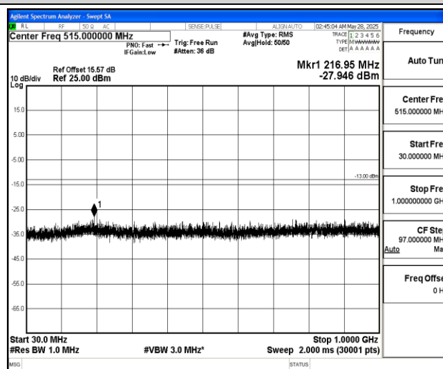
Band4-20MHz-QPSK-20050-1-0-Low-30-1000--27.95-PASS
