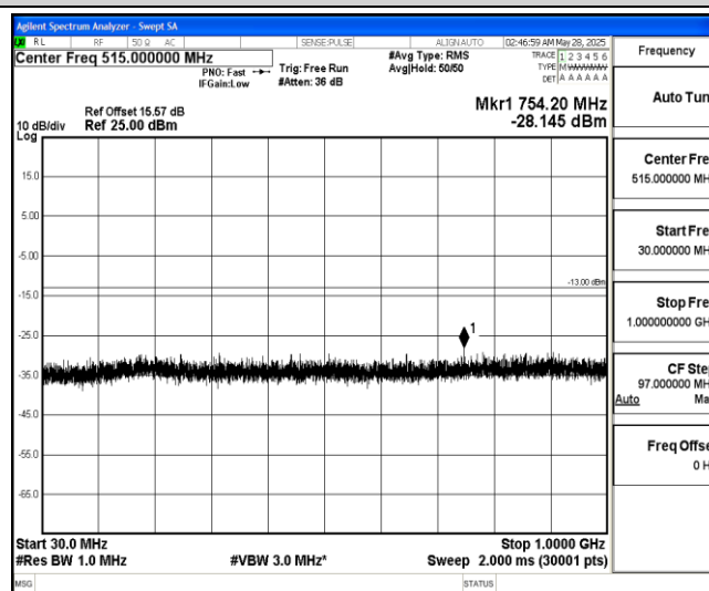
Band4-20MHz-16QAM-20050-1-0-Low-30-1000--28.15-PASS
