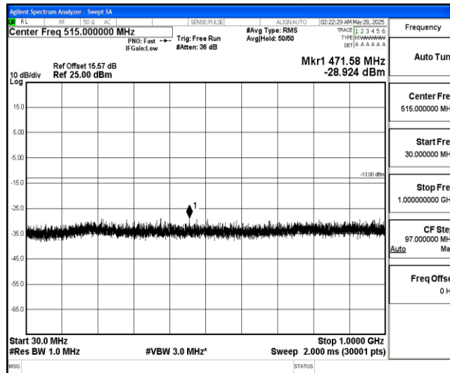
Band4-15MHz-QPSK-20175-1-0-Low-30-1000--28.92-PASS
