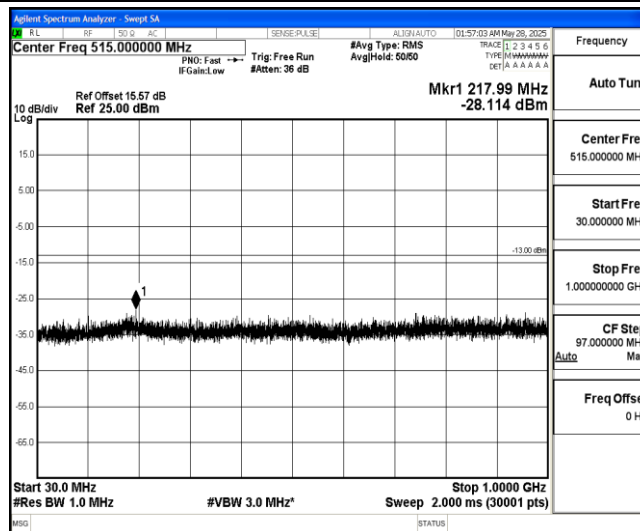
Band4-10MHz-QPSK-20175-1-0-Low-30-1000--28.11-PASS
