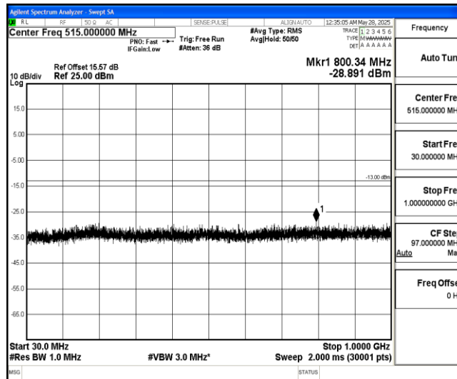
Band4-1.4MHz-QPSK-20175-1-0-Low-30-1000--28.89-PASS
