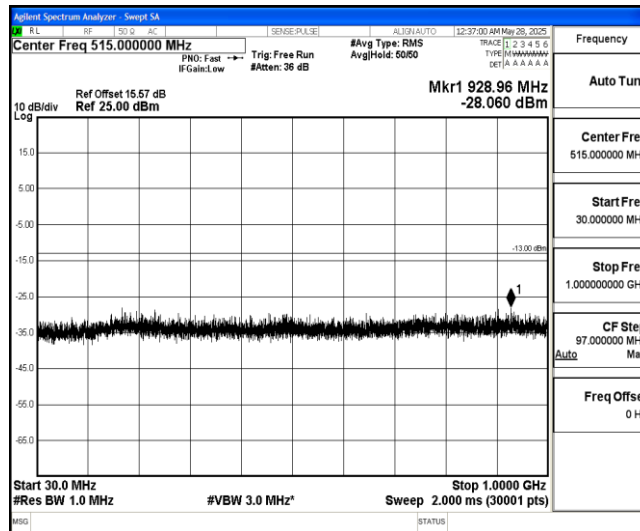
Band4-1.4MHz-16QAM-20175-1-0-Low-30-1000--28.06-PASS
