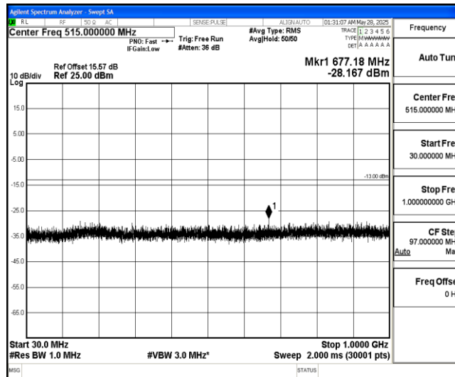
Band4-5MHz-QPSK-20175-1-0-Low-30-1000--28.17-PASS
