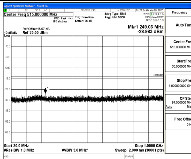
Band4-5MHz-QPSK-19975-1-0-Low-30-1000--28.98-PASS
