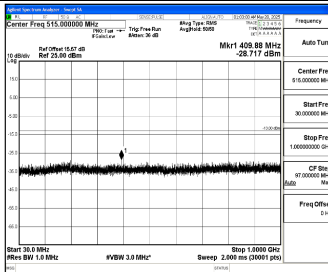
Band4-3MHz-QPSK-20175-1-0-Low-30-1000--28.72-PASS
