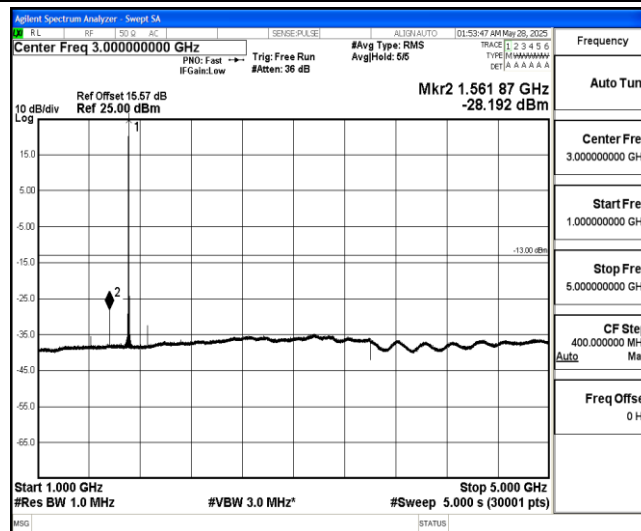
Band4-10MHz-QPSK-20000-1-0-Low-1000-5000--28.19-PASS
