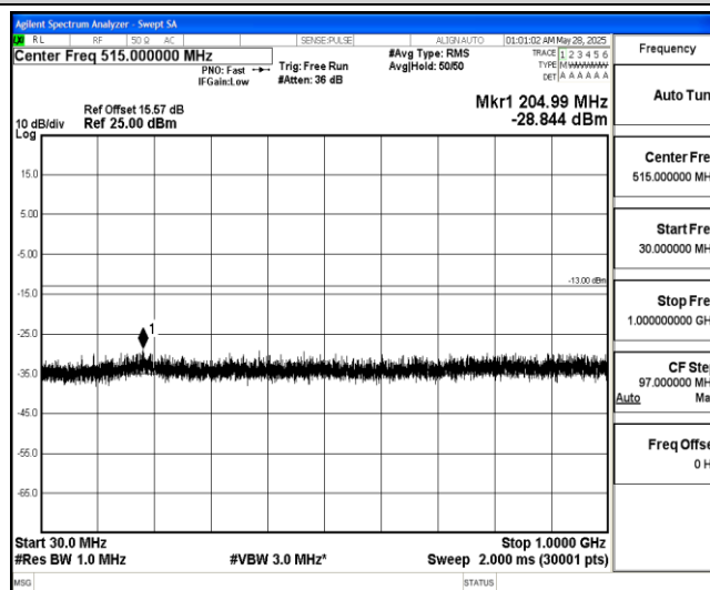
Band4-3MHz-16QAM-19965-1-0-Low-30-1000--28.84-PASS
