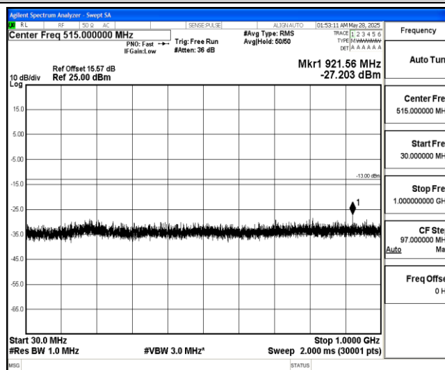
Band4-10MHz-QPSK-20000-1-0-Low-30-1000--27.2-PASS
