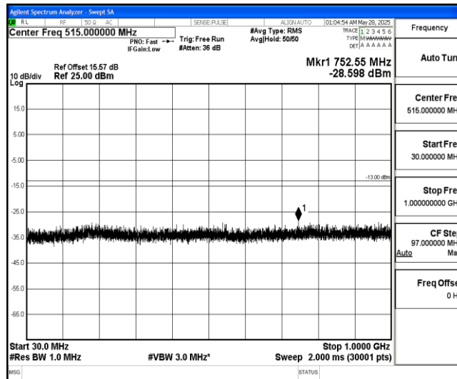
Band4-3MHz-16QAM-20175-1-0-Low-30-1000--28.6-PASS
