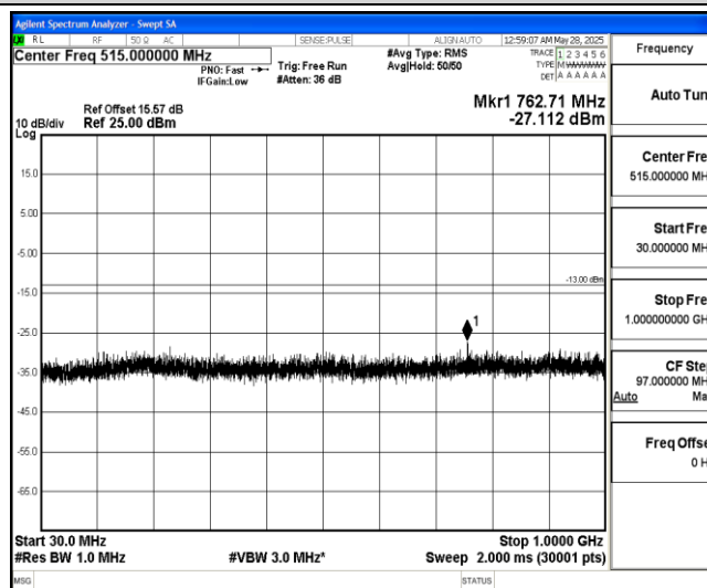
Band4-3MHz-QPSK-19965-1-0-Low-30-1000--27.11-PASS
