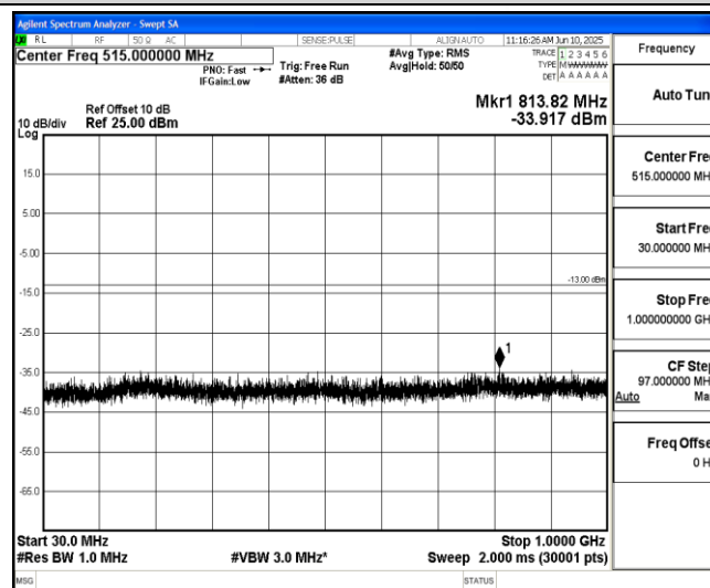
Band2-3MHz-QPSK-18900-1-0-Low-30-1000--33.92-PASS
