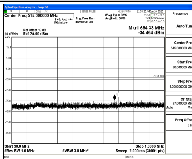
Band2-5MHz-QPSK-18900-1-0-Low-30-1000--34.46-PASS
