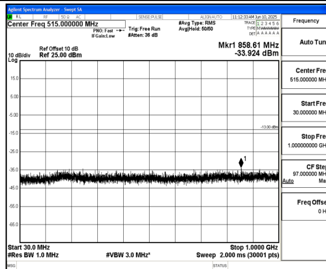
Band2-3MHz-QPSK-18615-1-0-Low-30-1000--33.92-PASS
