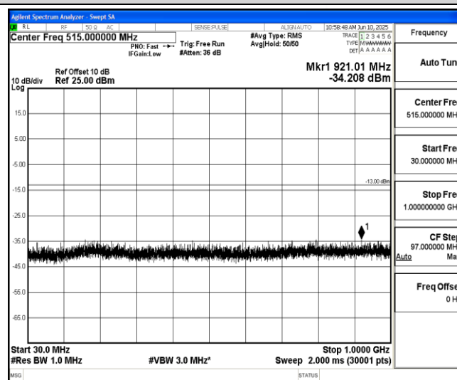
Band2-1.4MHz-QPSK-18900-1-0-Low-30-1000--34.21-PASS
