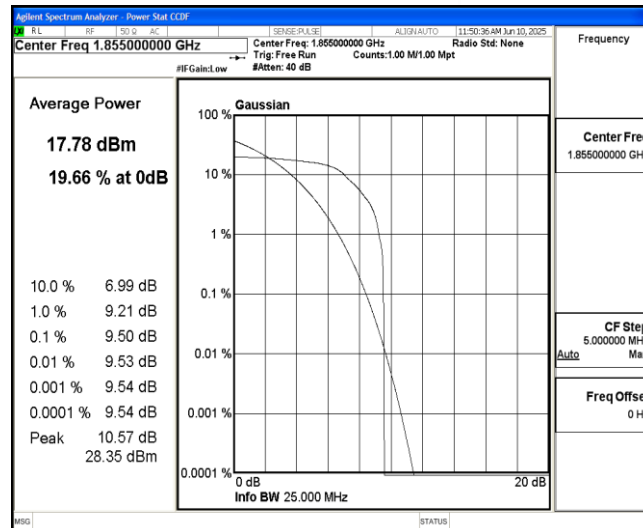
Band2-10MHz-QPSK-18650-1-0-Low-9.50-&lt;=13-PASS
