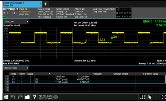
IEEE 802.11n 20MHz Channel 1
